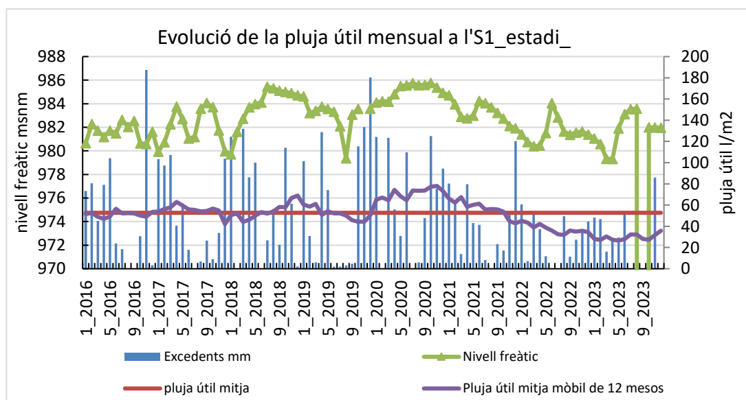
Figura 13. Evolució mensual dels nivells de l'S1 i dels excedents estimats (mitja país)
