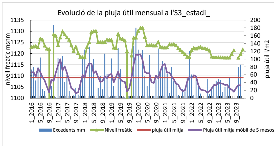
Figura 16. Evolució mensual dels nivells de l'S3 i dels excedents estimats (mitja país)
