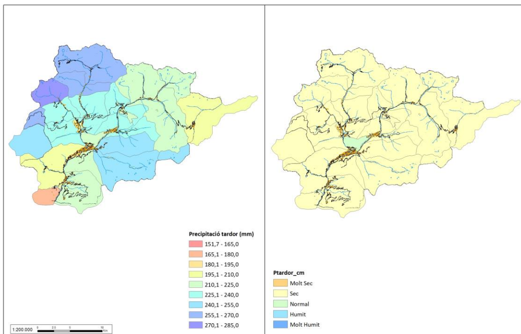
Figura 24. Mapa comparatiu de les precipitacions de la tardor del 2023 amb la mitjana climàtica 1981-2010 en les diferents unitats hidrogeològiques
