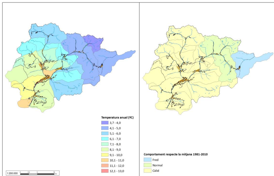
Figura 26. Mapa comparatiu de la temperatura del 2023 amb la mitjana climàtica 1981-2010 en les diferents unitats hidrogeològiques
