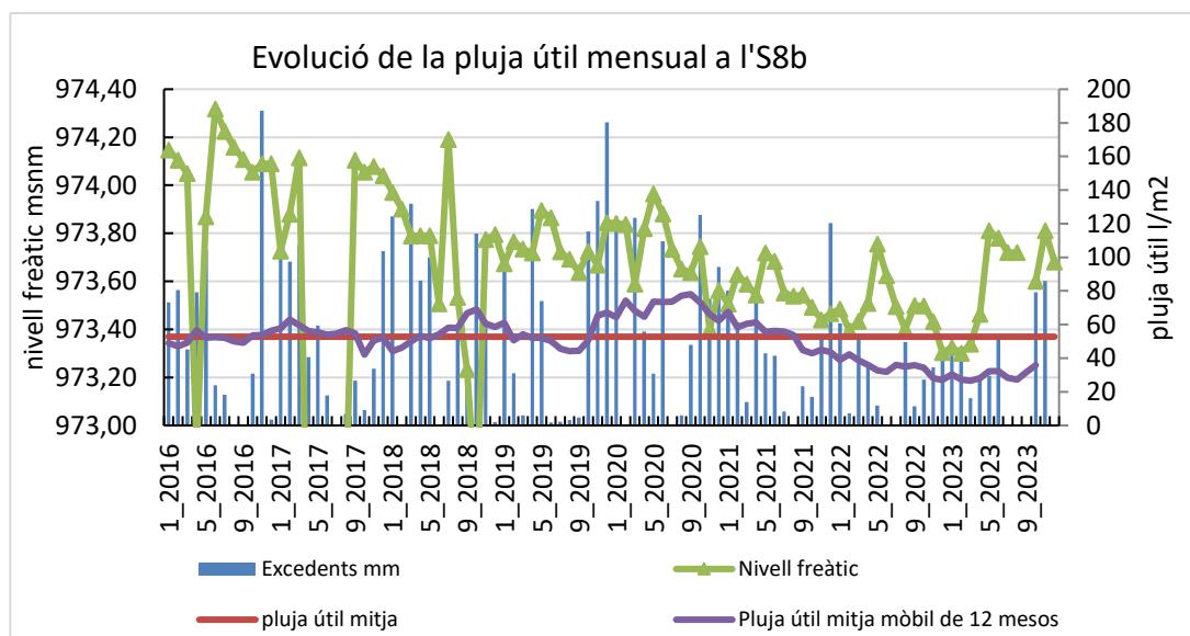
Figura 18. Evolució mensual dels nivells de l'S8b i dels excedents estimats (mitja país)
