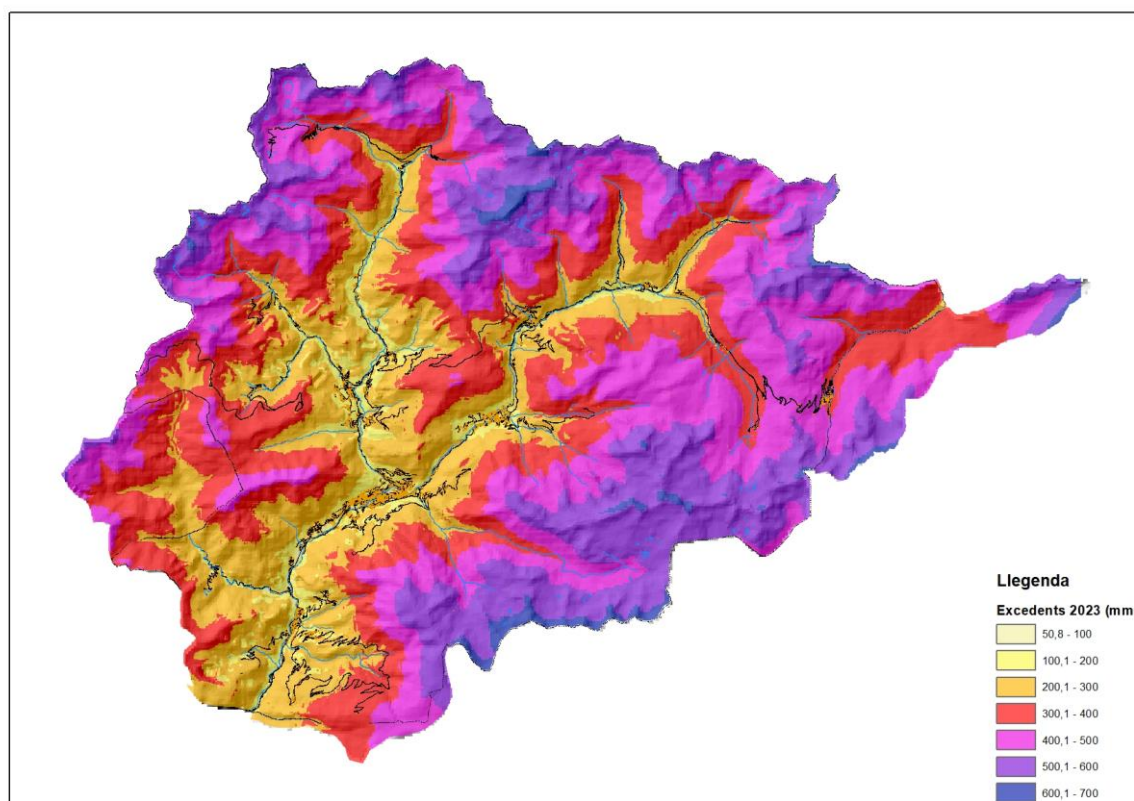
Figura 49. Mapa de distribució de la pluja útil o excedents estimats per l'any 2023
