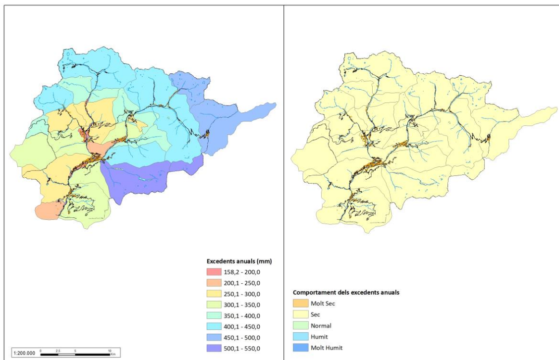
Figura 34. Mapa comparatiu dels excedents estimats del 2023 amb la mitjana climàtica 1981-2010 en les diferents unitats hidrogeològiques
