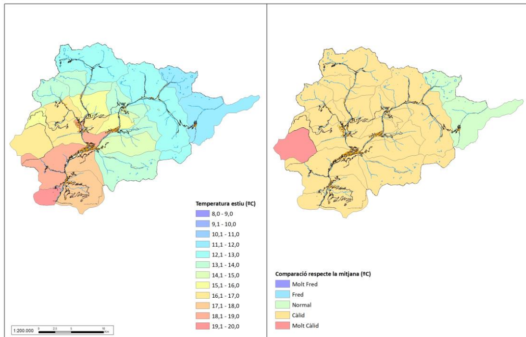
Figura 29. Mapa comparatiu de la temperatura de l'estiu del 2023 amb la mitjana climàtica 1981-2010 en les diferents unitats hidrogeològiques
