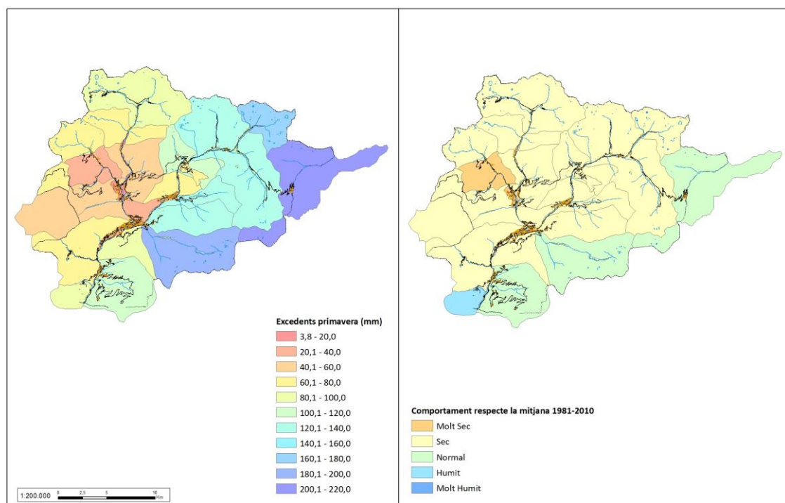
Figura 36. Mapa comparatiu dels excedents estimats a la primavera del 2023 amb la mitjana climàtica 1981-2010 en les diferents unitats hidrogeològiques
