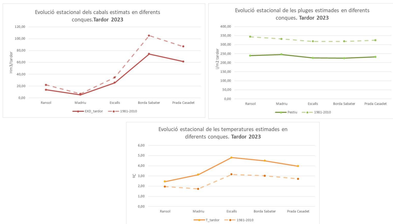
Figura 46. Anàlisi de la tardor dels cabals estimats, de les precipitacions i de la temperatura en les diferents conques.
