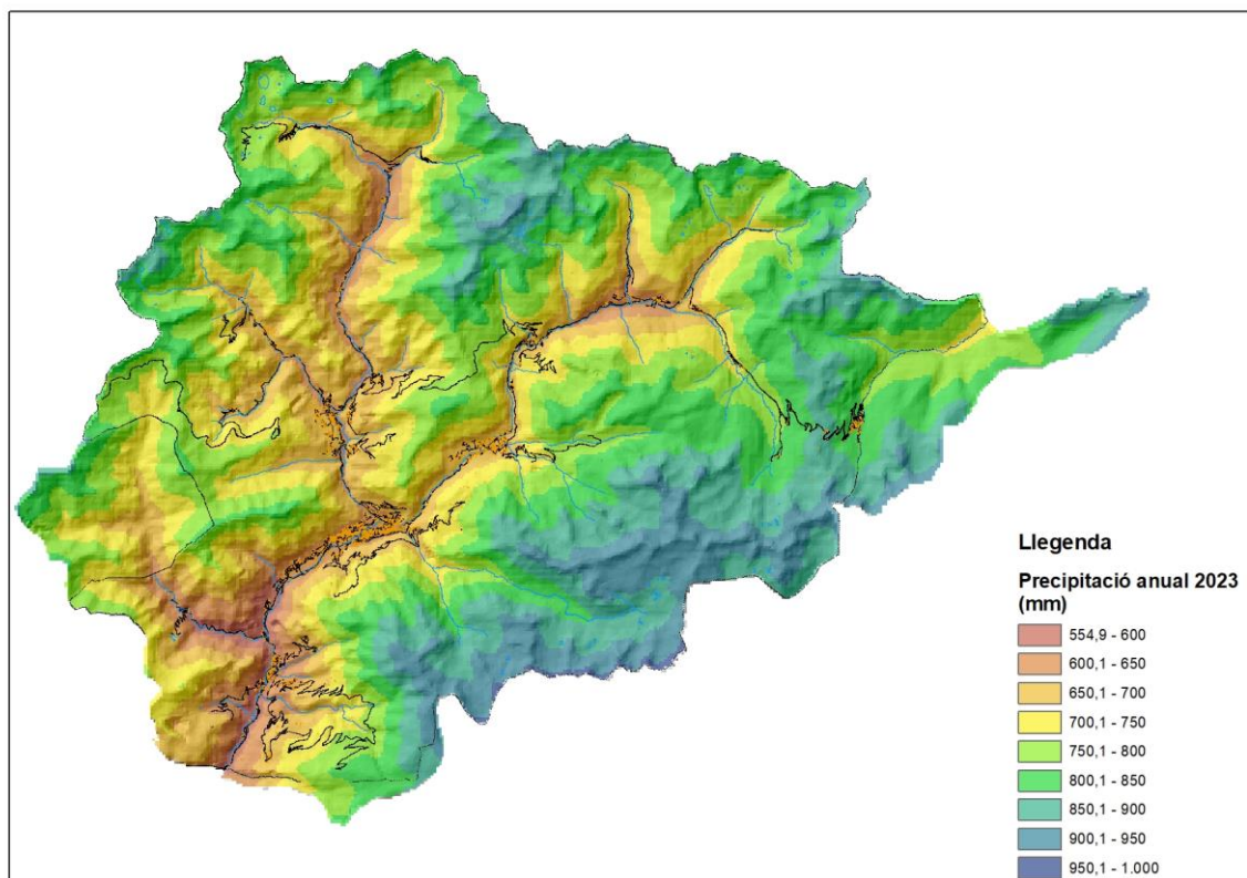
Figura 1. Mapa de distribució de les precipitacions acumulades el 2023. Dades base facilitades pel l'ARI
