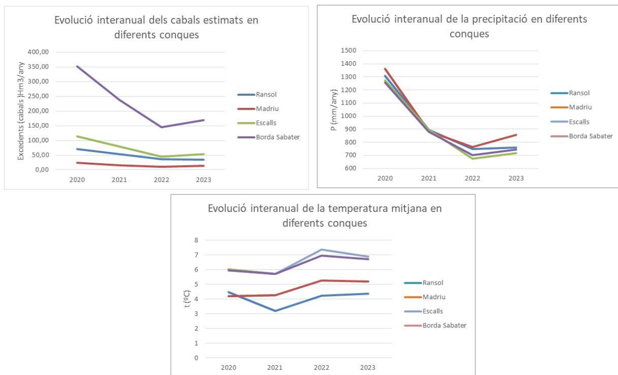
Figura 47. Evolució interanual de la precipitació, temperatura i excedents en les diferents conques
