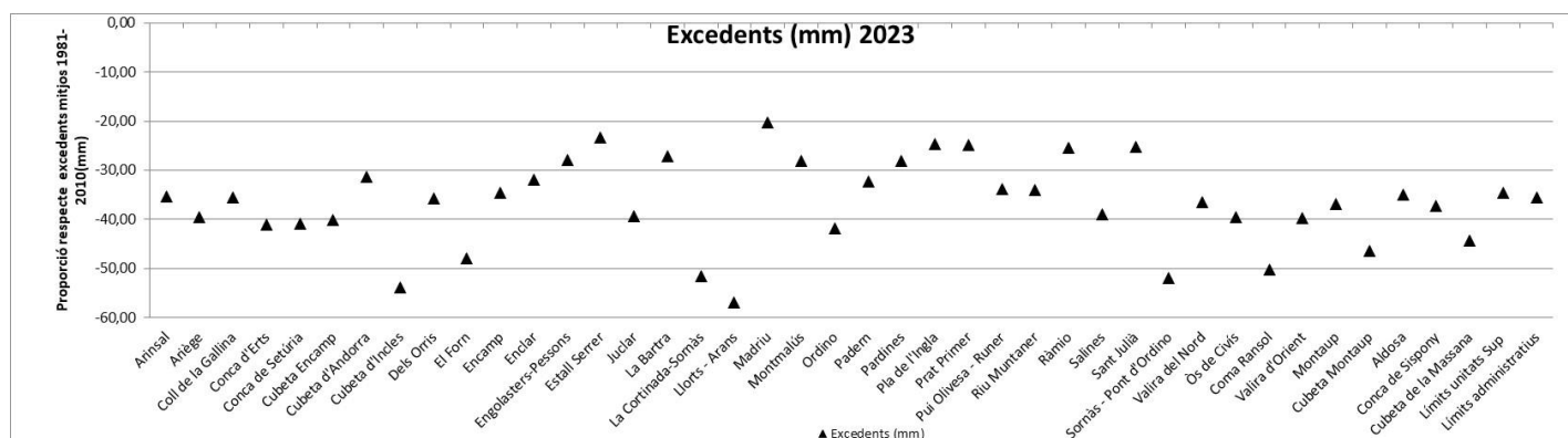
Figura 33. Gràfic de distribució dels excedents en les diferents unitats hidrogeològiques descrites en l'estudi del M.I. Govern, 2007. Si el valor mig representa el 100%, els valors del gràfic representen el percentatge per sobre o per sota la mitjana.
