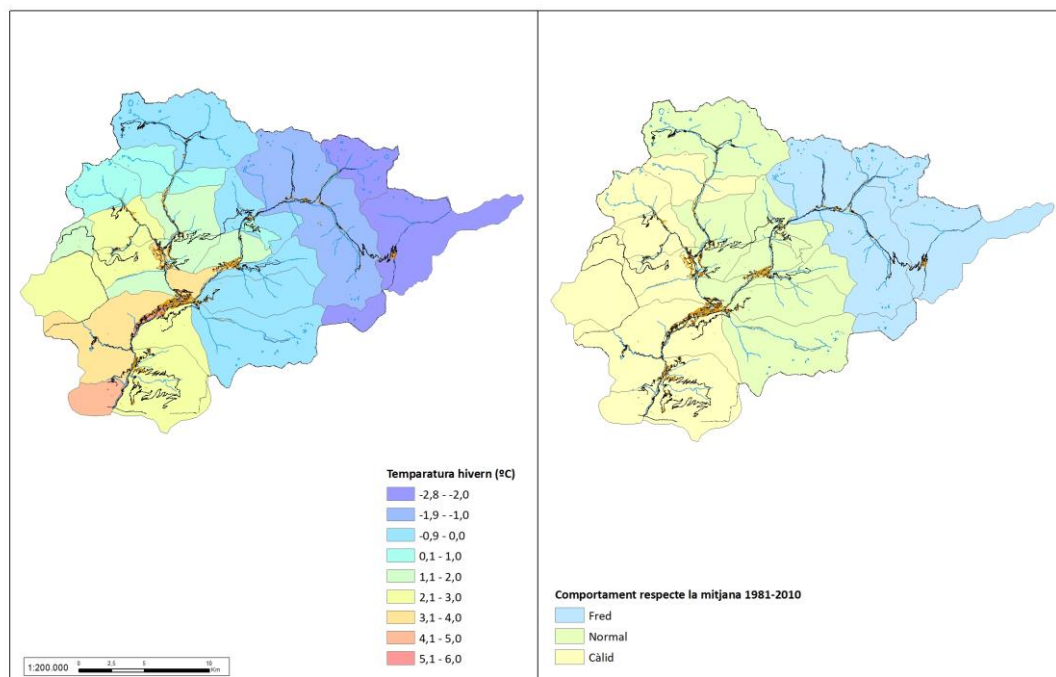
Figura 27. Mapa comparatiu de la temperatura de l'hivern del 2023 amb la mitjana climàtica 1981-2010 en les diferents unitats hidrogeològiques
