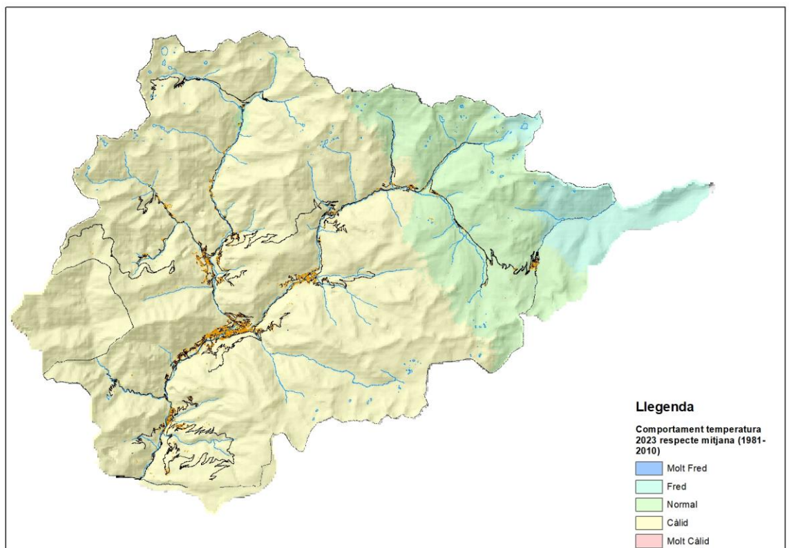
Figura 4. Mapa de les diferències de temperatura de l'any 2023 respecte la mitja.
