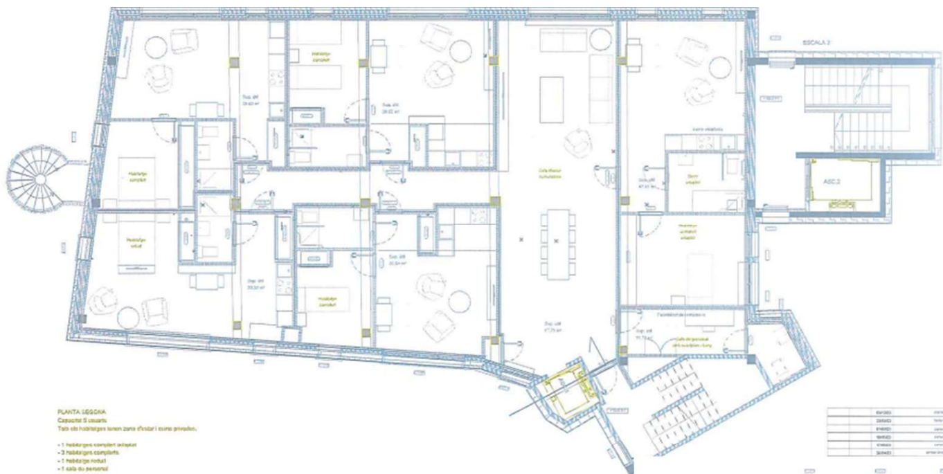
Planta segona
