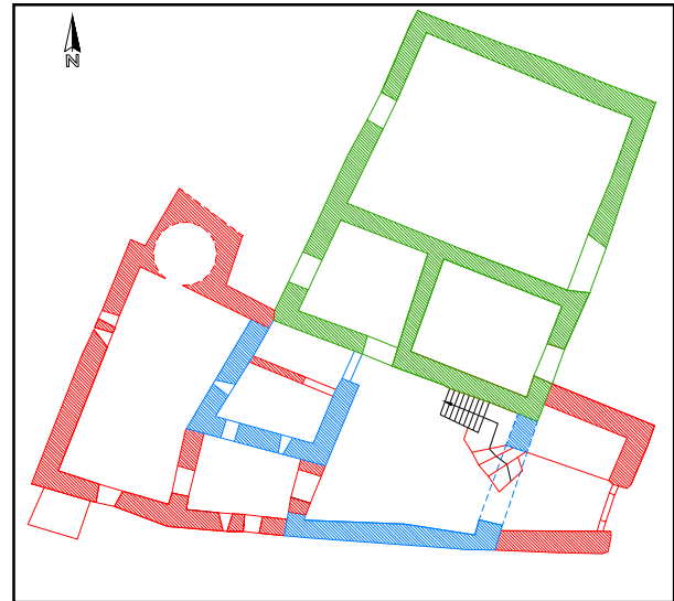
Vista de la planta baixa de Cal Ribot durant la fase III
