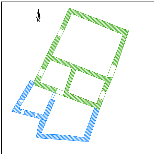
Vista de la planta baixa de Cal Ribot durant la fase II
