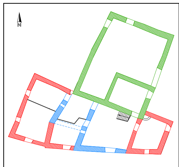
Vista de la primera planta de Cal Ribot durant la fase III
