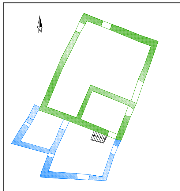
Vista de la primera planta de Cal Ribot durant la fase II
