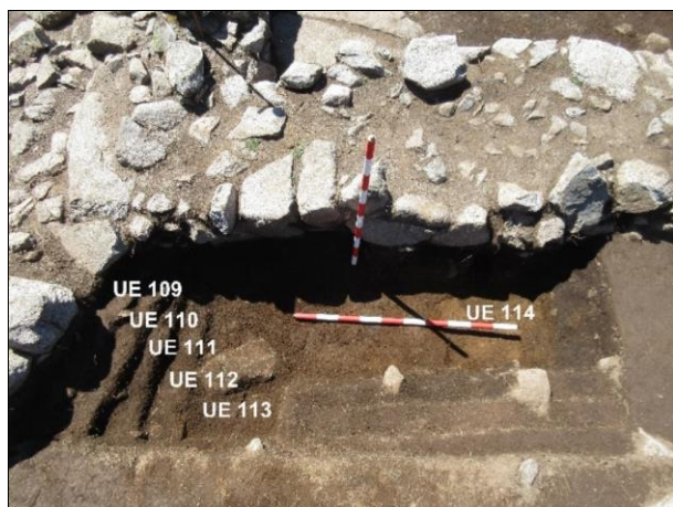
F. 33. Vista de la seqüència estratigràfica del Sondeig nord-est.
