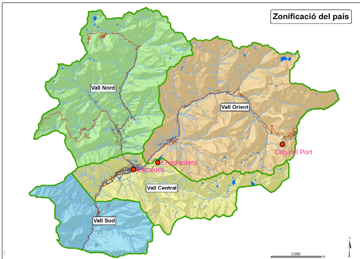
Mapa 2: Localització de les estacions automàtiques de mesurament d'ozó (any 2016).
