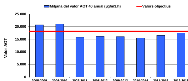
Gràfic 2: Evolució històrica del valor de l'AOT40.
