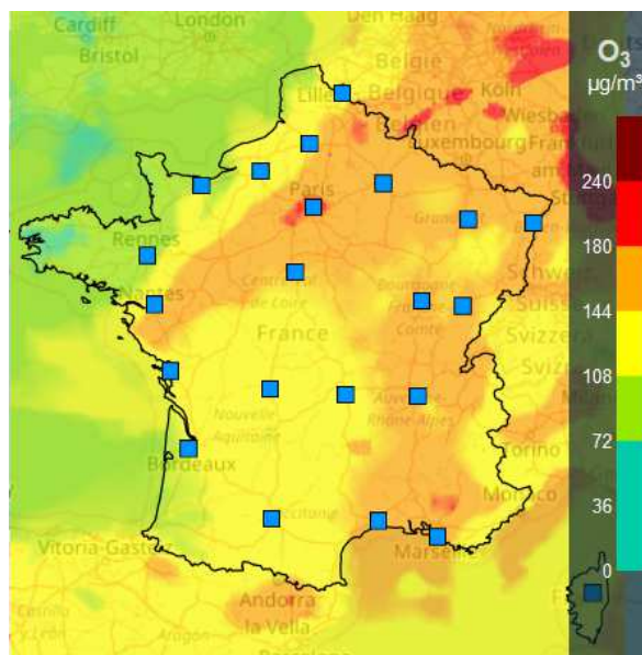
Mapa 3: Mapa de màxim diari pel programa PREV'AIR (26/08/2016).
