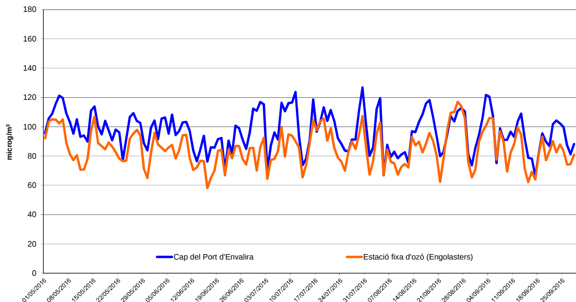
Gràfic 4: Evolució de les mitjanes horàries (de l'1 de maig del 2016 al 30 de setembre del 2016).
