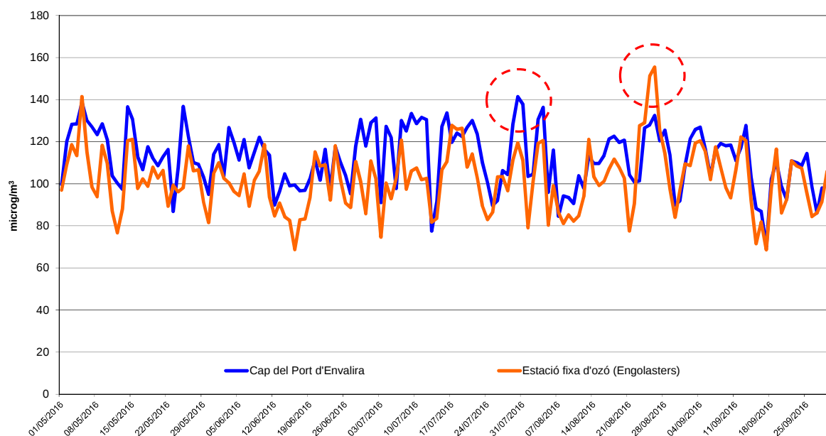
Gràfic 3: Evolució dels màxims horaris (de l'1 de maig del 2016 al 30 de setembre del 2016).
