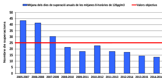
Gràfic 1: Evolució històrica del nombre de dies de superacions de 120 \mu\text{g}/\text{m}^3 .
