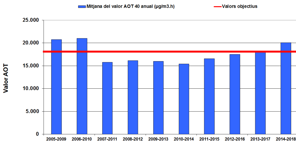
Gràfic 12: Evolució històrica dels valors de l'AOT 40.
