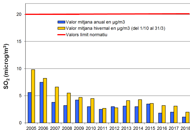
Gràfic 6: Mitjana d'SO 2 els darrers anys.
