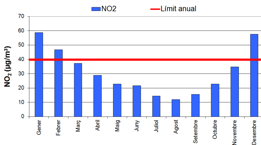
Gràfic 13: Evolució estacional de l' \text{NO}_2 a la vall central (any 2018).
