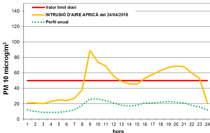
Gràfic 15: Perfils diaris de partícules PM10 a la vall central.
