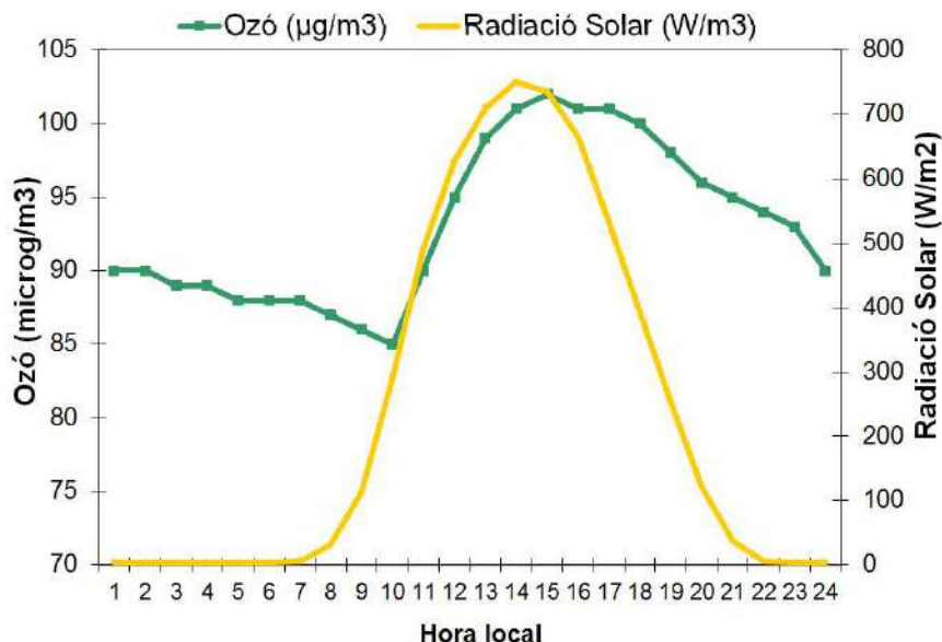
Gràfic 16: Perfil diari de l'ozó en el periurbà de la vall central (any 2018).
