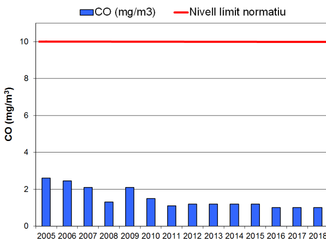
Gràfic 7: Evolució dels màxims de les mitjanes octohoràries.
