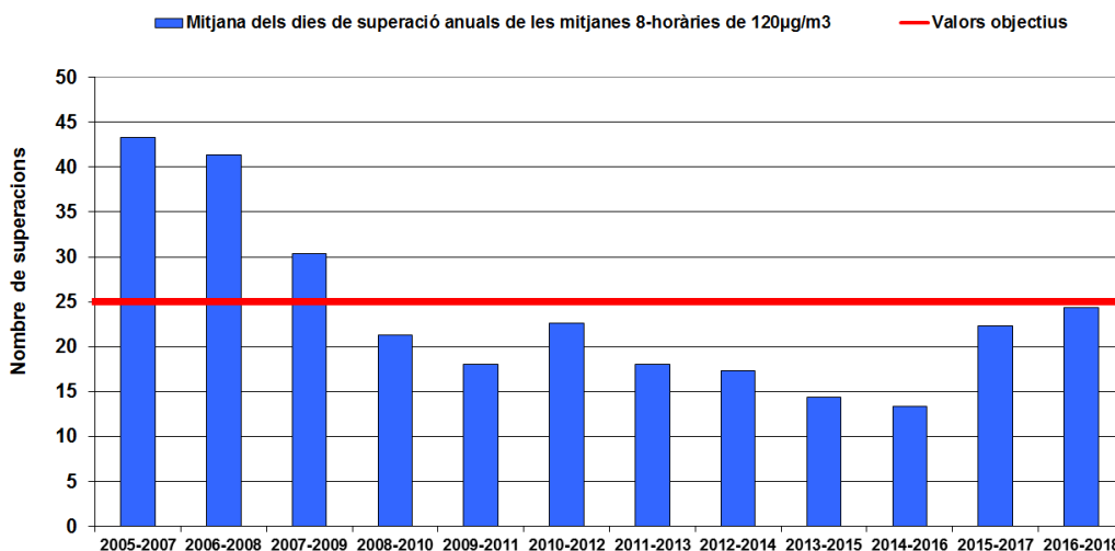
Gràfic 11: Evolució històrica del nombre de dies de superacions de 120 µg/m 3 .
