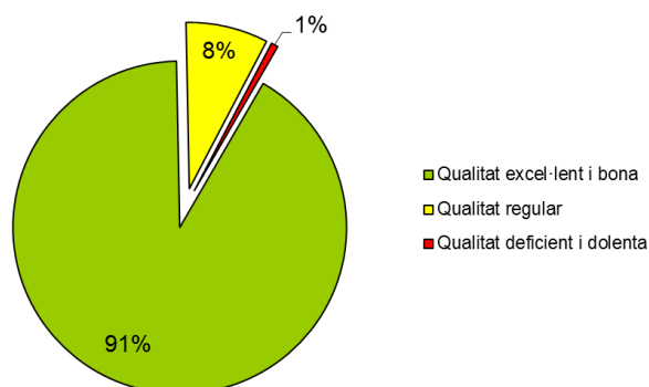
Gràfic 2: Índex de qualitat de l'aire (IQA) – Any 2017
