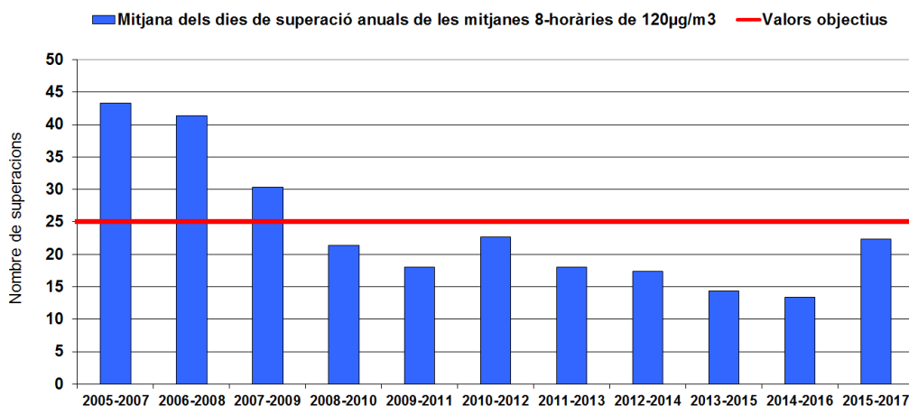
Gràfic 11: Evolució històrica del nombre de dies de superacions de 120 µg/m 3 .
