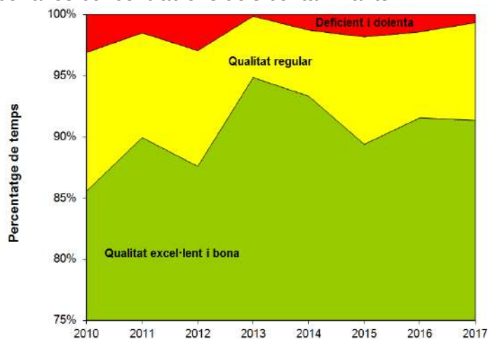
Gràfic 3: Evolució de l'IQA des de l'any 2010
