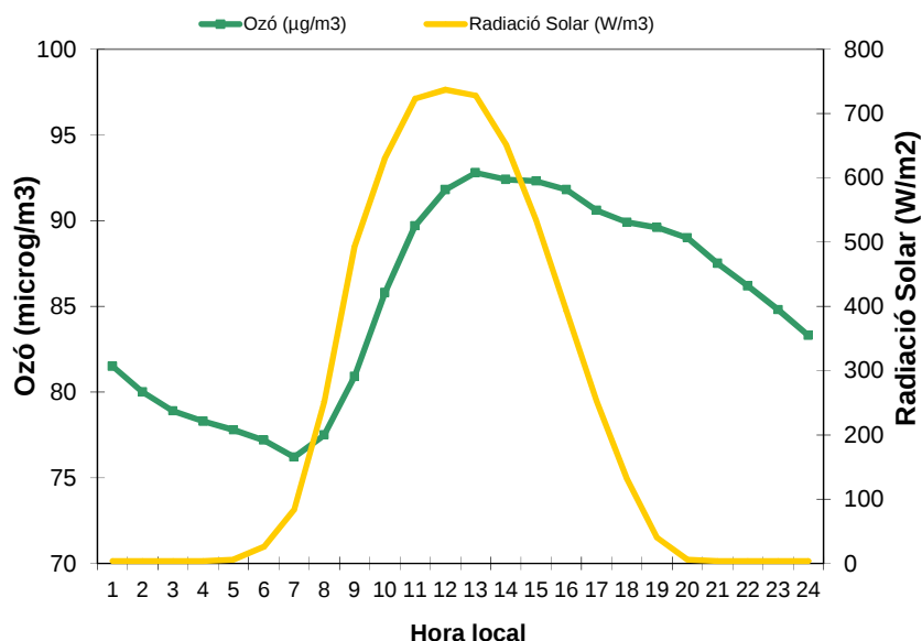
Gràfic 16: Perfil diari de l'ozó en el periurbà de la vall central (any 2017).
