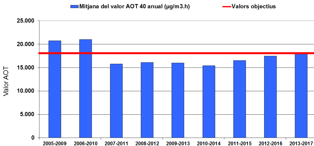
Gràfic 12: Evolució històrica dels valors de l'AOT 40.
