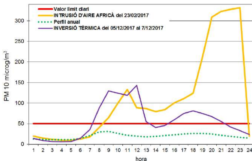
Gràfic 15: Exemples de 2 perfils diaris de partícules PM10 a la vall central.
