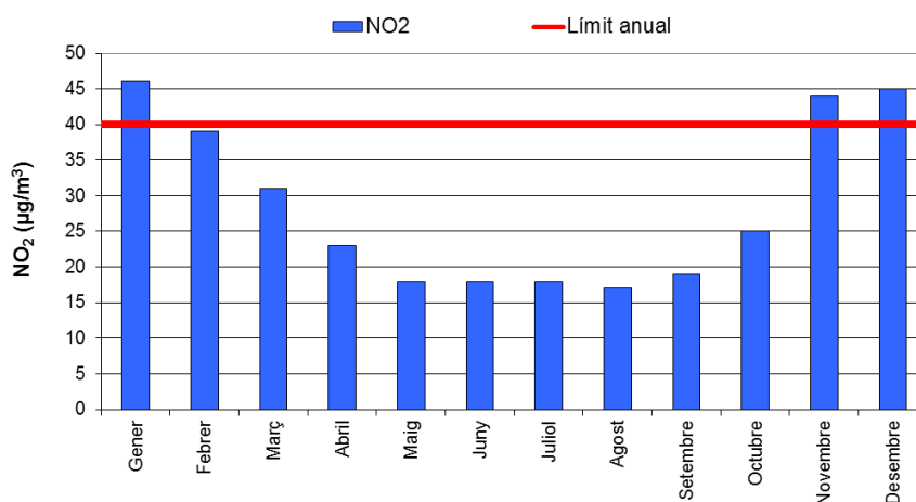
Gràfic 13: Evolució estacional de l' \text{NO}_2 a la vall central (any 2017).
