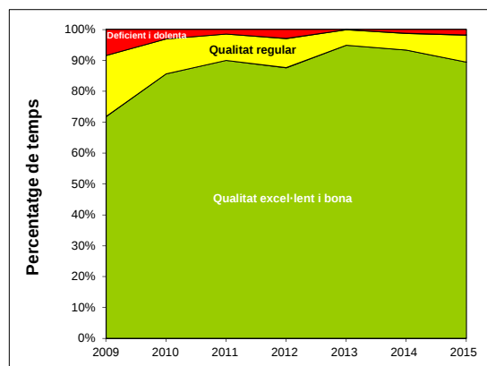
Gràfic 2: Evolució de l'IQA
