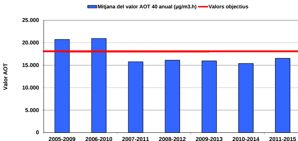
Gràfic 13: Evolució històrica dels valors de l'AOT 40.
