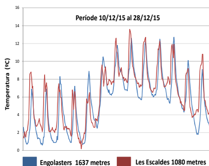
Gràfic 1: Inversió tèrmica a la vall central.
