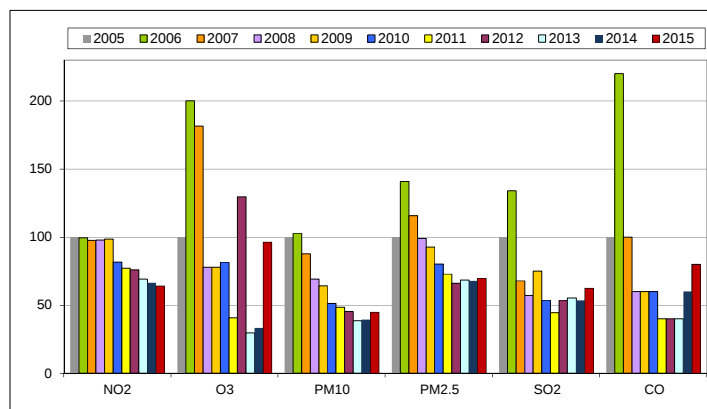
Gràfic 3: Evolució dels contaminants des del 2005
