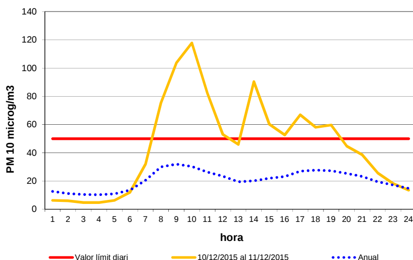
Gràfic 16: Exemples de perfil diari de partícules PM10 a la vall central.
