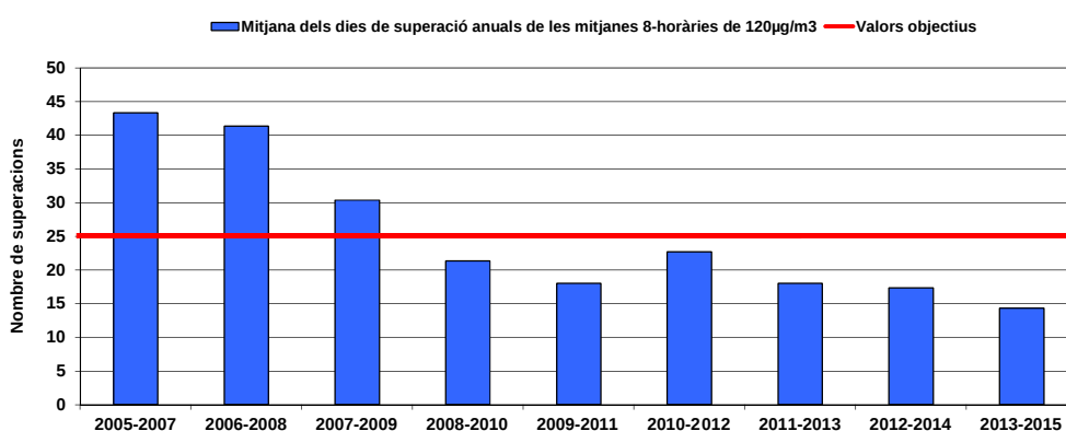
Gràfic 12: Evolució històrica del nombre de dies de superacions de 120 \mu\text{g}/\text{m}^3 .
