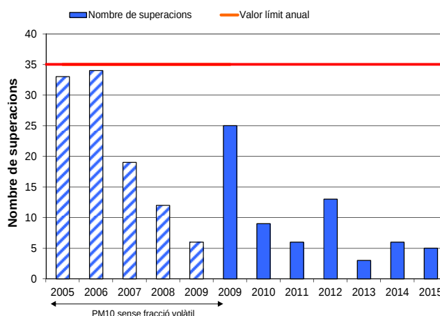
Gràfic 10: Evolució del nombre de superacions diàries.
