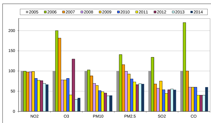
Gràfic 3: Evolució dels contaminants des del 2005
