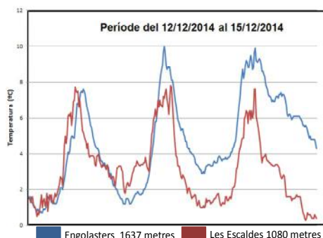
Gràfic 1: Inversió tèrmica a la vall central.
