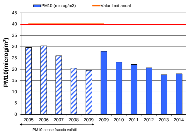
Gràfic 9: Evolució de la mitjana anual de PM10.
