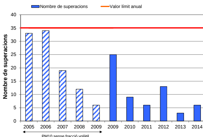
Gràfic 10: Evolució del nombre de superacions diàries.
