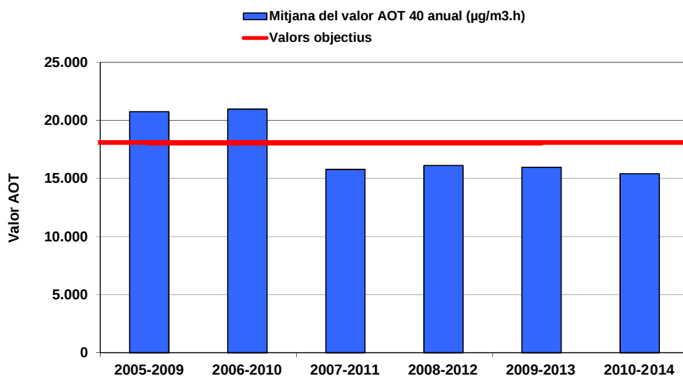
Gràfic 13: Evolució històrica dels valors de l'AOT 40.
