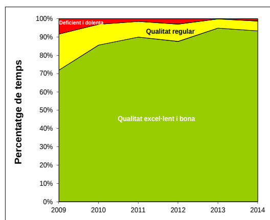
Gràfic 2: Evolució de l'IQA
