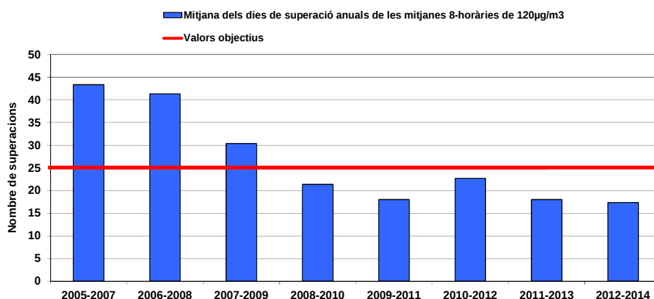
Gràfic 12: Evolució històrica del nombre de dies de superacions de 120 \mu\text{g}/\text{m}^3 .
