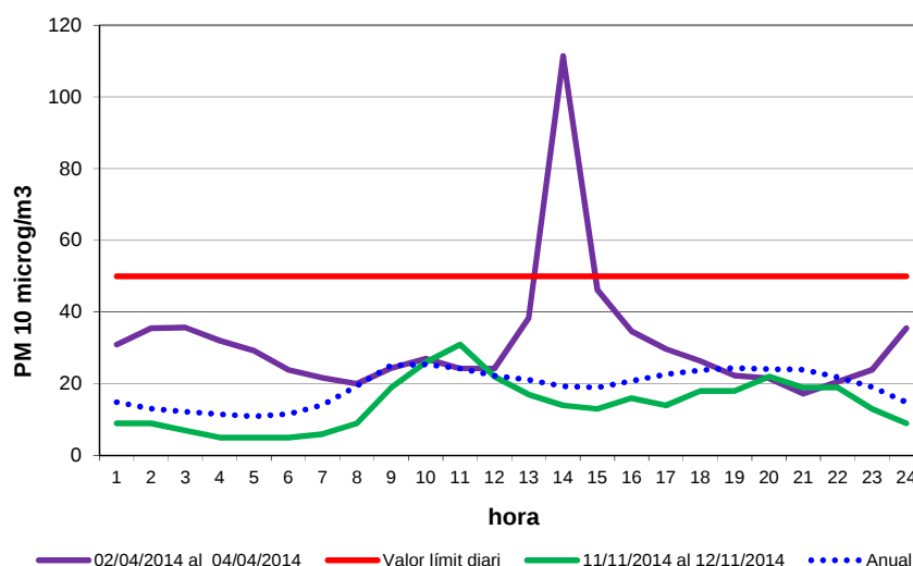
Gràfic 16: Exemples de perfil diari de partícules PM10 a la vall central.
