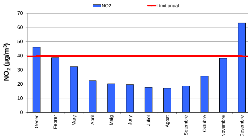
Gràfic 14: Evolució estacional de l' \text{NO}_2 a la vall central.
