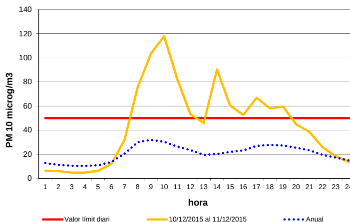
Gràfic 42: Exemples de perfil diari de partícules PM10 a la vall central.
