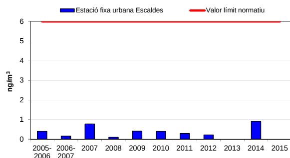
Gràfic 28: Evolució de l'arsènic (període 2005-2015)
