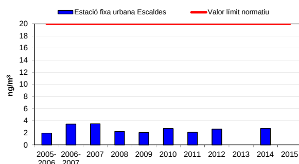
Gràfic 30: Evolució del níquel (període 2005-2015)
