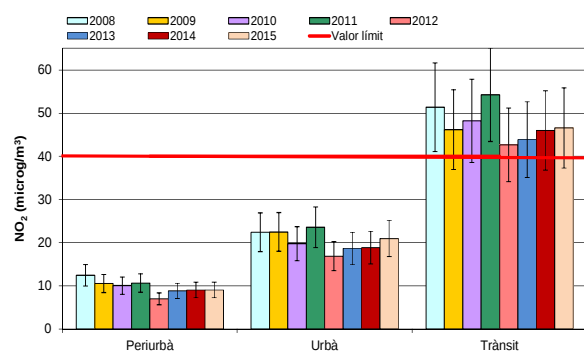
Gràfic 9: Evolució del NO 2 per àmbits
