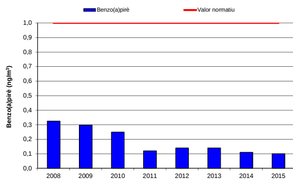
Gràfic 38: Evolució del benzo (A) pirè. Anys 2008 a 2015
