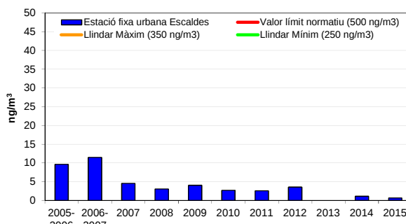
Gràfic 31: Evolució del plom (període 2005-2015)
