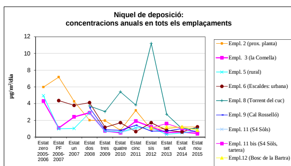
Gràfic 34: Evolució del níquel en diferents àmbits de mesura
