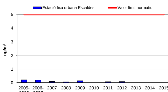
Gràfic 29: Evolució del cadmi (període 2005-2015)
