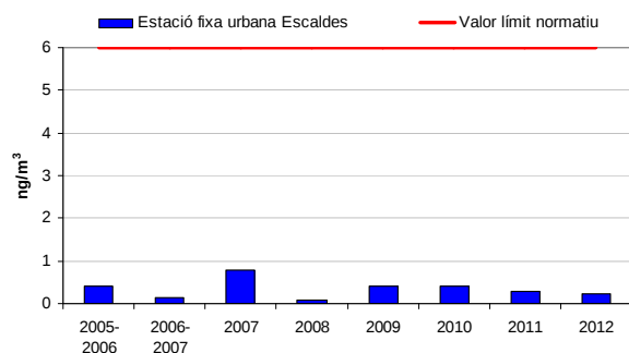
Gràfic 30: Evolució de l'arsènic (període 2005-2012)
