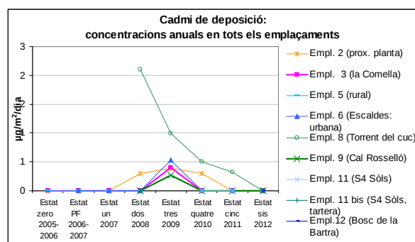
Gràfic 35: Evolució del cadmi en diferents àmbits de mesura
