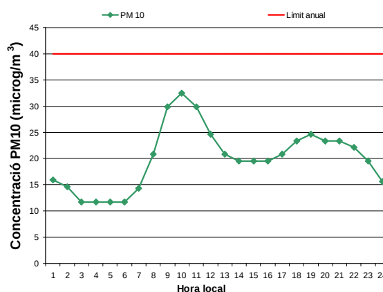
Gràfic 45: Perfil diari de PM10 a la vall central.
