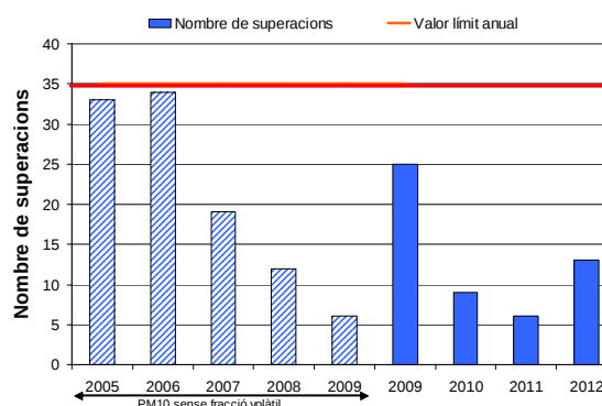
Gràfic 20: Evolució del nombre de superacions diàries
