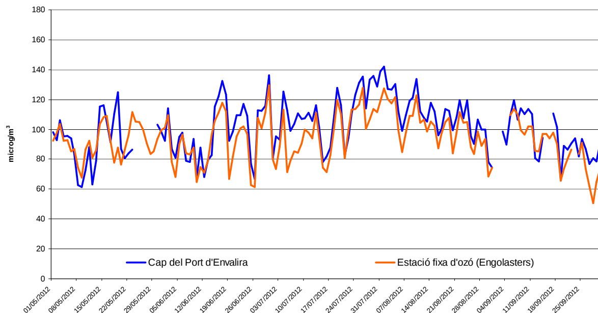
Gràfic 25: Evolució de la mitjana diària (de l'1 de maig del 2012 al 30 de setembre del 2012).
