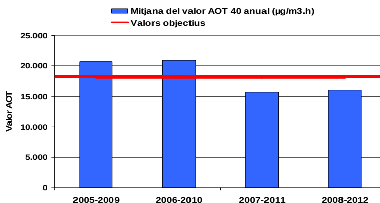
Gràfic 23: Evolució històrica dels valors de l'AOT 40
