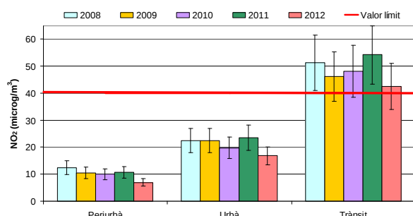
Gràfic 9: Evolució del NO 2 per àmbits
