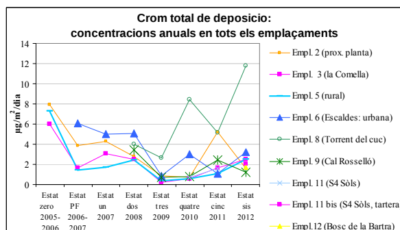
Gràfic 39: Evolució del crom total en diferents àmbits de mesura
