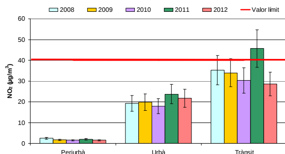
Gràfic 11: Evolució del NO 2 per àmbits
