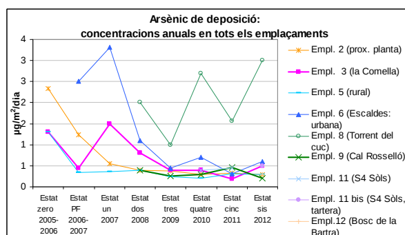
Gràfic 34: Evolució de l'arsènic en diferents àmbits de mesura
