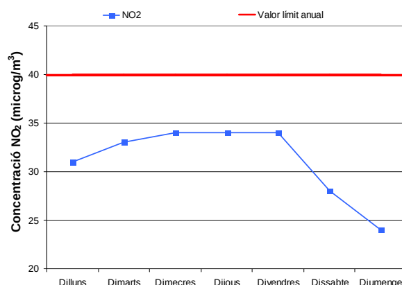
Gràfic 44: Perfil setmanal del NO 2 a la vall central.
