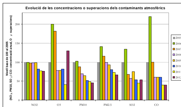
Gràfic 2: Evolució dels contaminants des del 2005.
