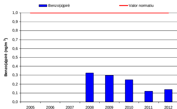
Gràfic 41: Evolutiu del benzo (A) pirè. Anys 2008 a 2012
