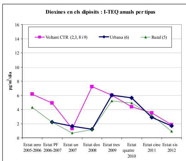
Gràfic 40: Evolució de les dioxines i furans en deposició
