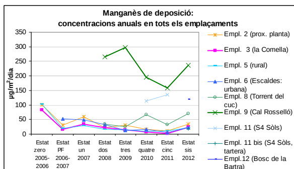
Gràfic 38: Evolució del manganès en diferents àmbits de mesura
