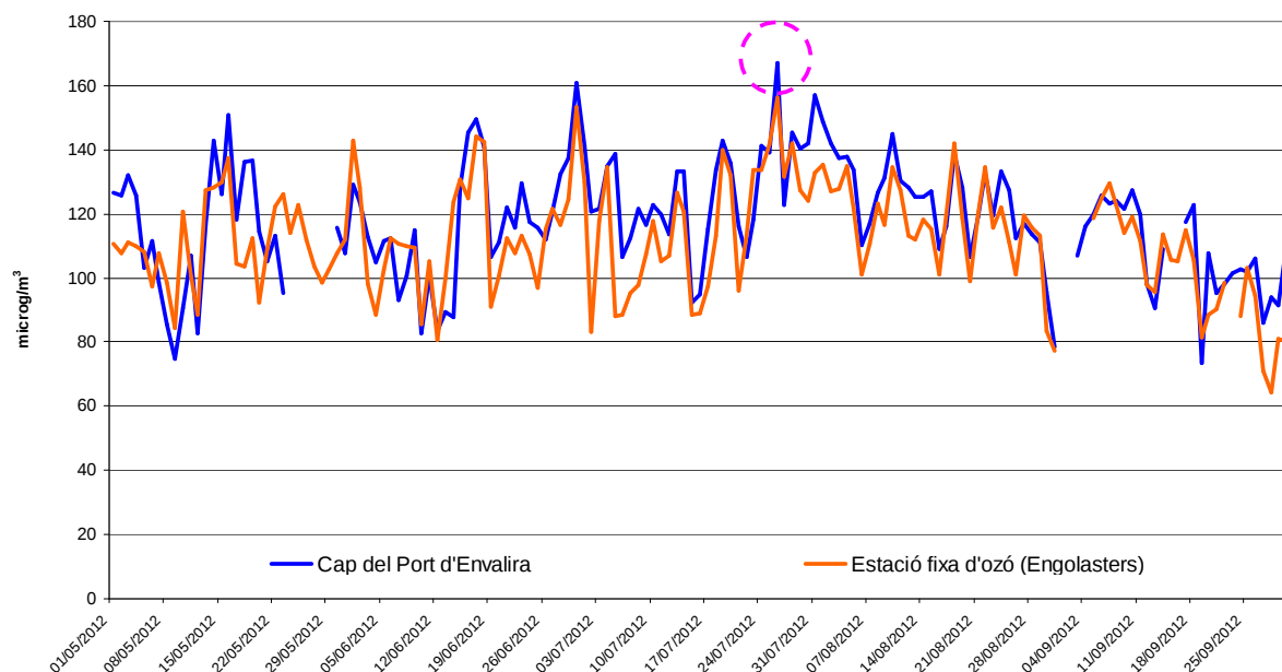
Gràfic 24: Evolució dels màxims diaris (de l'1 de maig del 2012 al 30 de setembre del 2012).
