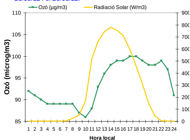
Gràfic 47: Perfil diari de l'ozó en el periurbà de la vall central.
