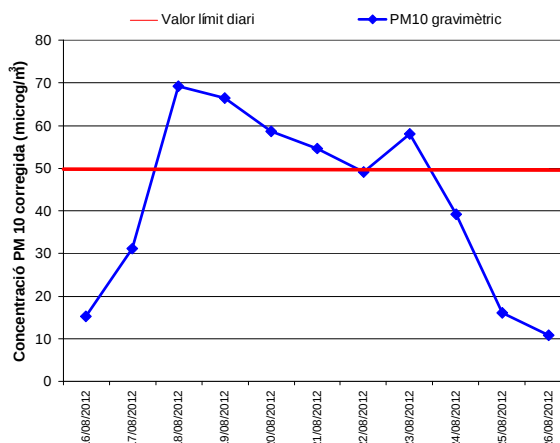
Gràfic 46: Nivells diaris de PM10 a la vall central entre el 16/08/12 i el 26/08/12.
