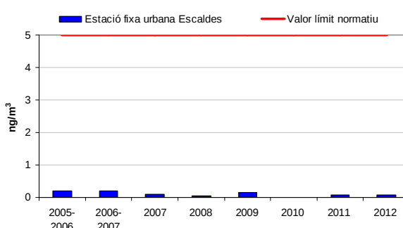
Gràfic 31: Evolució del cadmi (període 2005-2012)
