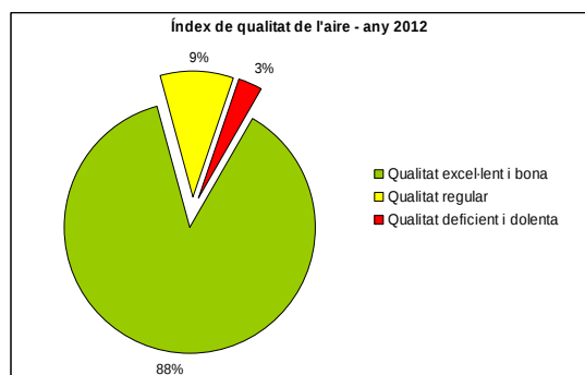
Gràfic 1: Resultats del 2012 de l'IQA.
