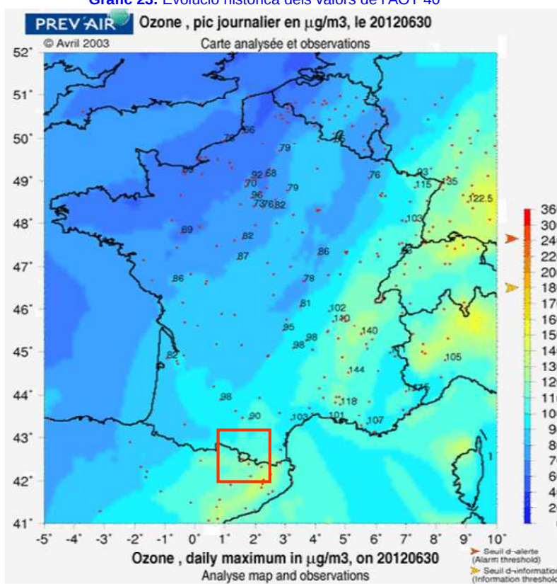
Mapa 3: Mapa analitzat pel programa PREV'AIR (30/06).
