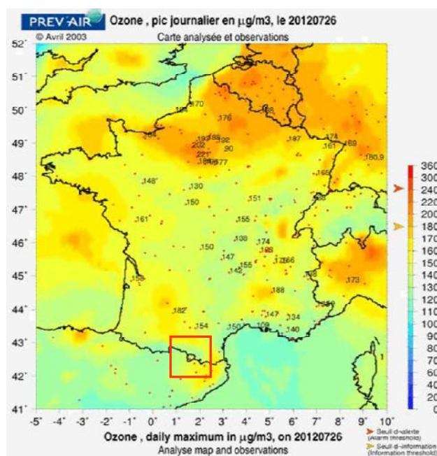
Mapa 5: Mapa analitzat pel programa PREV'AIR (26/07).
