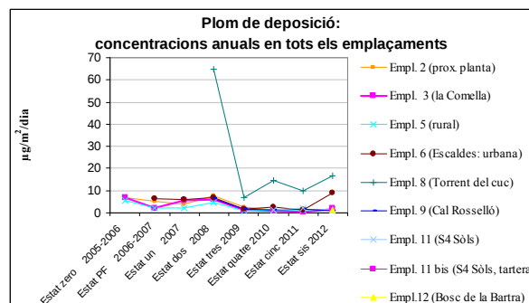
Gràfic 37: Evolució del plom en diferents àmbits de mesura
