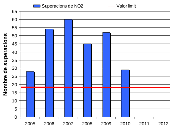
Gràfic 4: Evolució del nombre de superacions del límit horari objectiu per al 2010 de 200 \mu\text{g}/\text{m}^3 de \text{NO}_2
