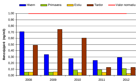
Gràfic 42: Evolutiu estacional del benzo (A) pirè
