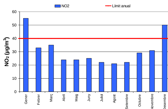
Gràfic 43: Evolució estacional del NO 2 a la vall central.
