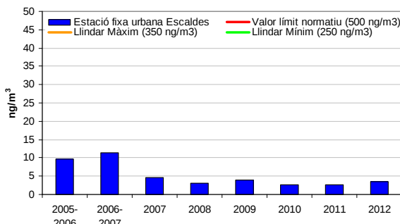
Gràfic 33: Evolució del plom (període 2005-2012)
