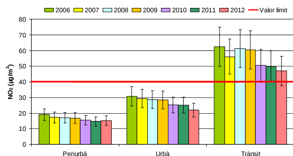
Gràfic 10: Evolució del NO 2 per àmbits
