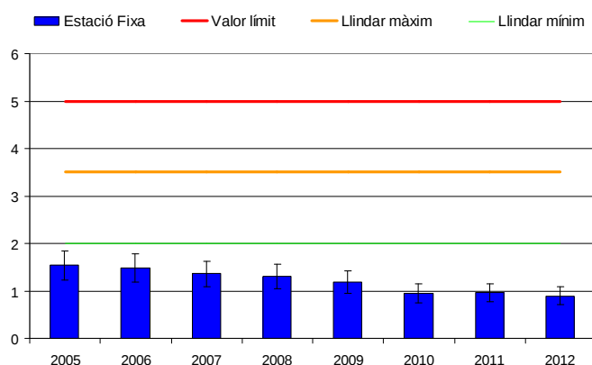
Gràfic 29: Nivells globals de benzè a l'estació de referència urbana
