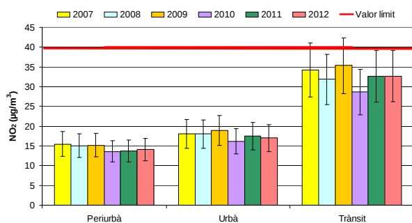
Gràfic 12: Evolució del NO 2 per àmbits
