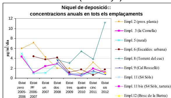
Gràfic 36: Evolució del níquel en diferents àmbits de mesura
