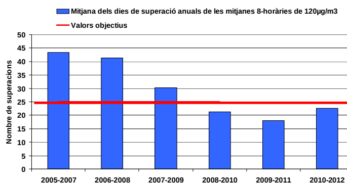
Gràfic 22: Evolució històrica del nombre de dies de superacions de 120\mu\text{g}/\text{m}^3
