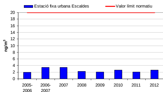
Gràfic 32: Evolució del níquel (període 2005-2012)
