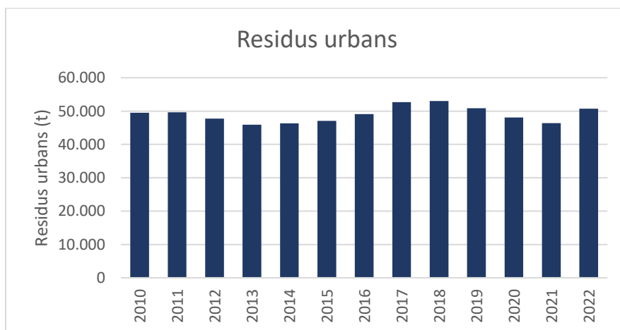
Gràfic 3. Evolució dels residus urbans (segons la definició de la Directiva 2018/851)
