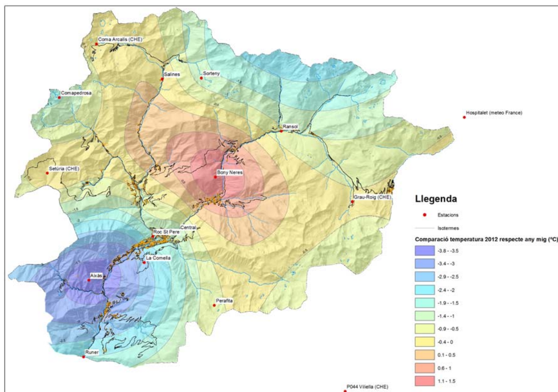
Figura 6. Mapa de les diferències de temperatura de l'any 2012 respecte la mitja.
