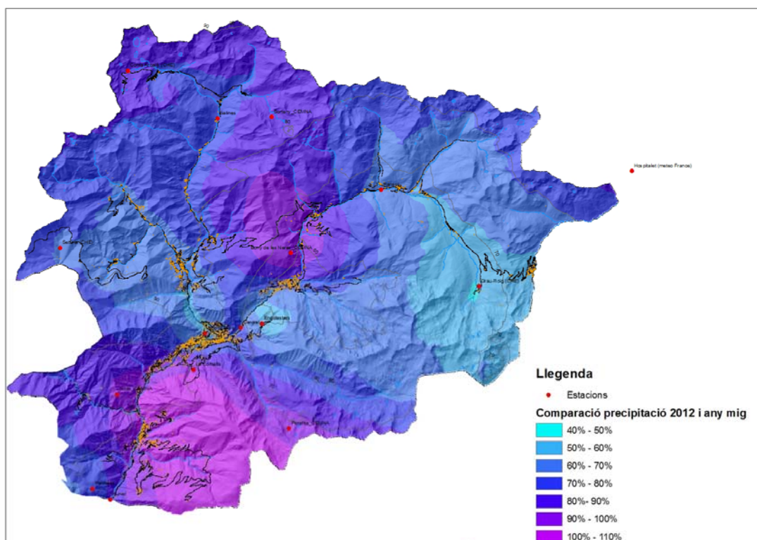
Figura 3. Mapa comparatiu de les quantitats acumulades registrades el 2012 i els corresponents valors mitjans.
