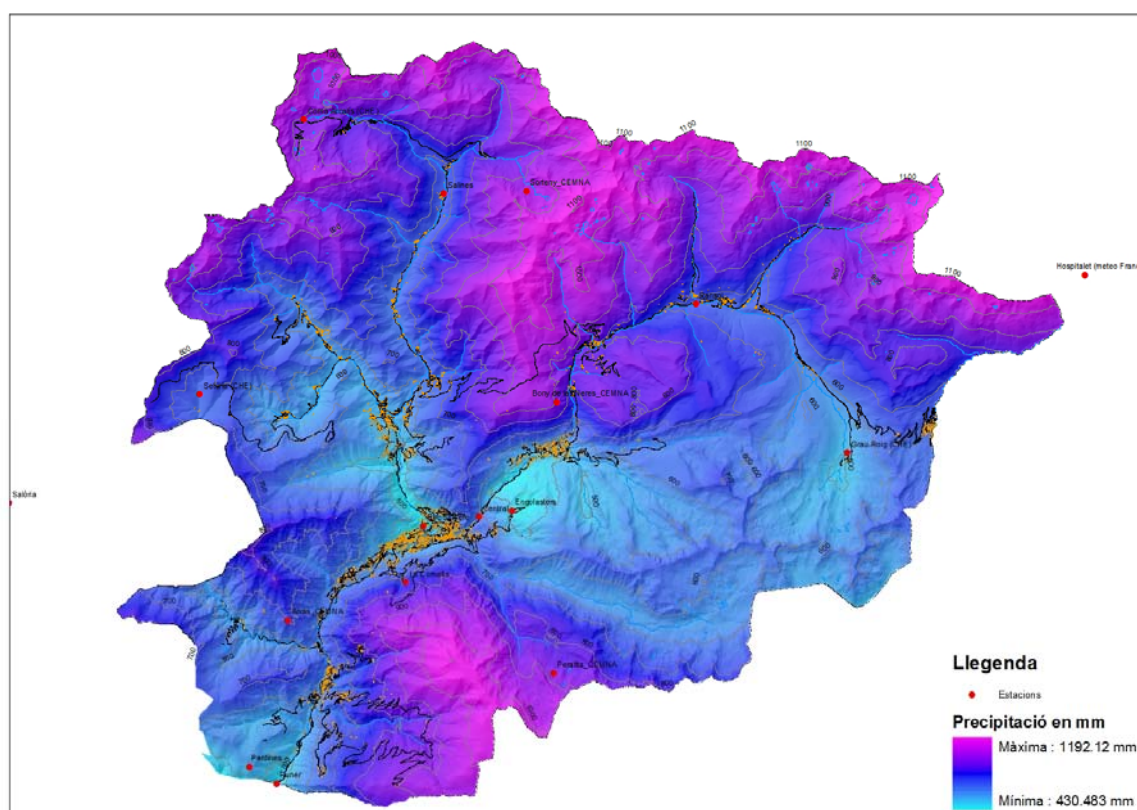
Figura 2. Mapa d'isoietes de les precipitacions acumulades el 2012.
