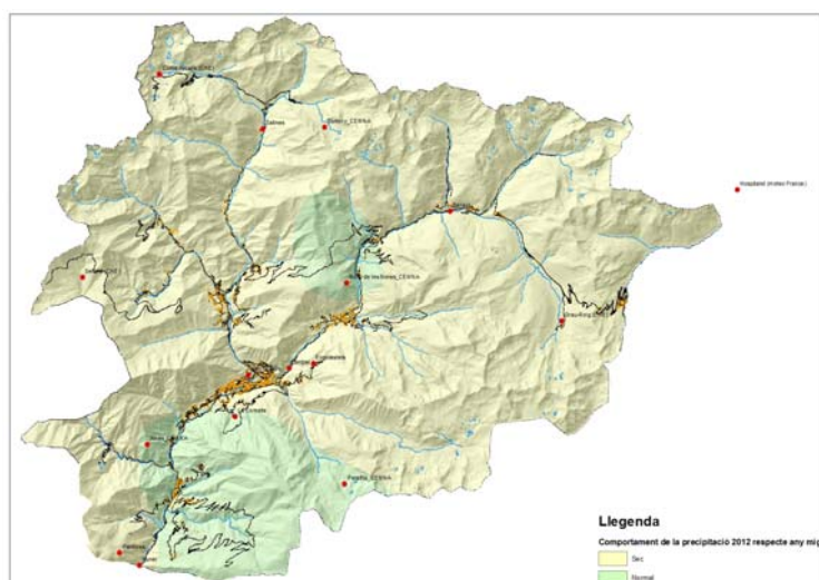
Figura 4. Mapa de distribució de la valoració de les precipitacions de l'any 2012 respecte la mitjana
