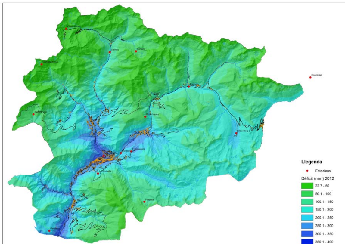
Figura 19. Mapa de distribució dels dèficits estimats per l'any 2012. R=30 mm seguint el mètode de Thornthwaite. El mètode de càlcul ha consistit en la diferència entre ETP i ETR quan no hi ha reserva disponible.
