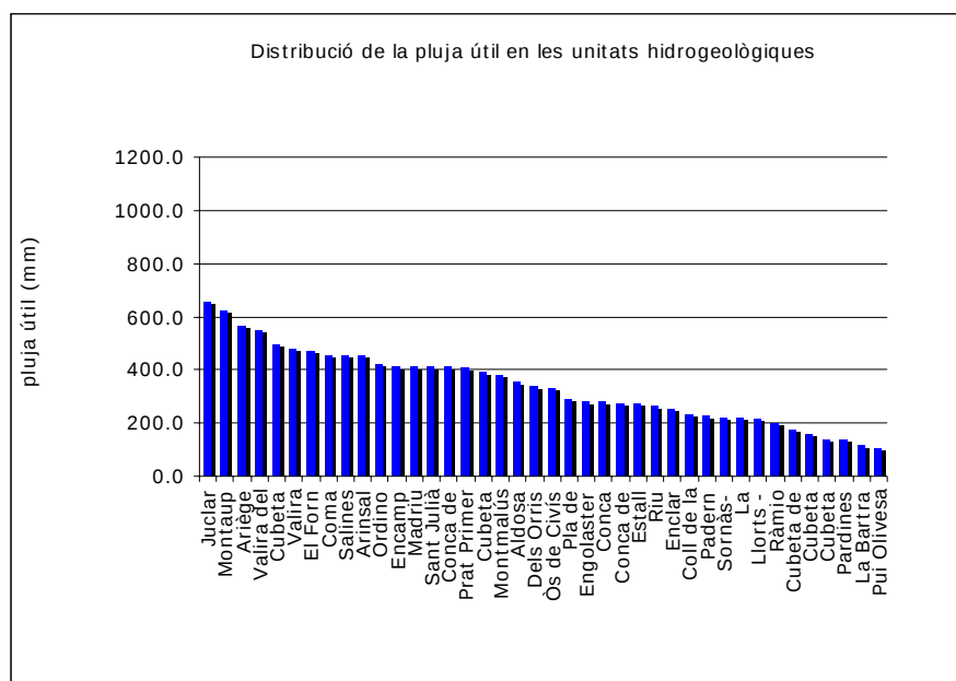
Figura 15. Gràfic de distribució de la Pluja útil
