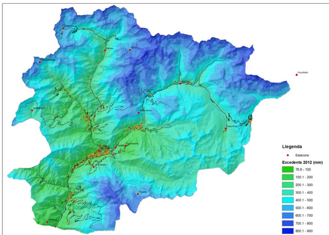
Figura 18. Mapa de distribució de la pluja útil o excedents estimats per l'any 2012. R \leq 30 mm seguint el mètode de Thornthwaite
