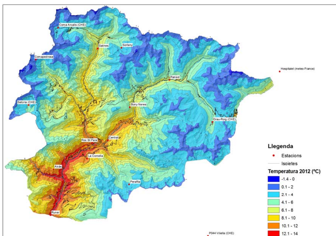
Figura 5. Mapa de distribució de les temperatures mitges del 2012
