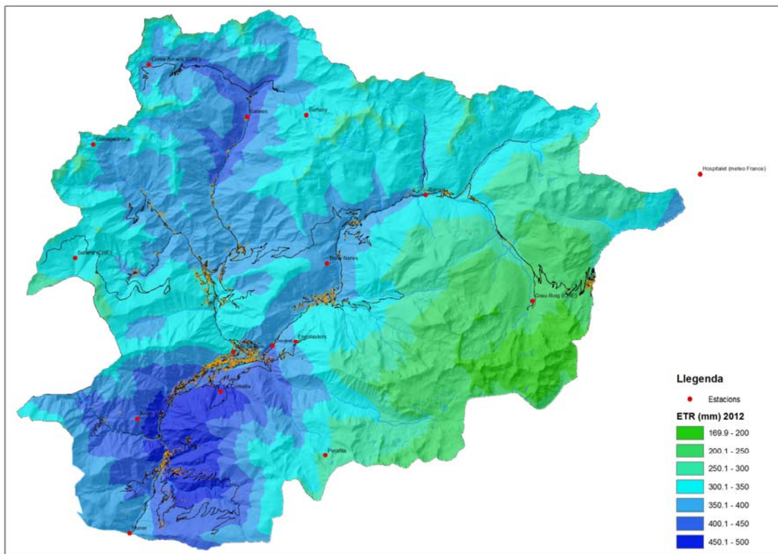
Figura 17. Mapa de distribució de l'ETR estimada per l'any 2012, segons el mètode de Thornthwaite.
