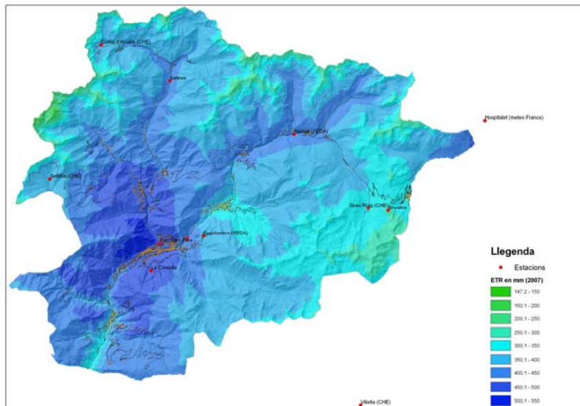
Figura 17. Mapa de distribució de l'ETR estimada per l'any 2007, segons el mètode de Thornthwaite.
