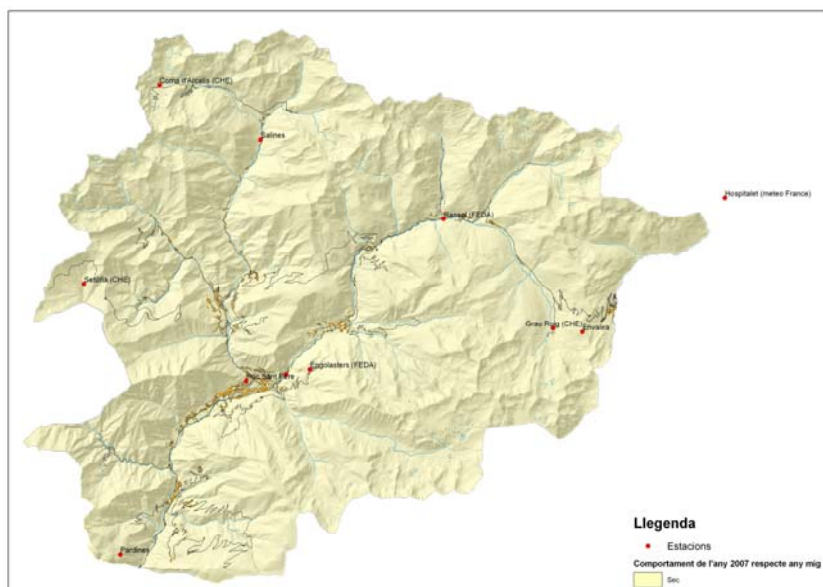
Figura 4. Mapa de distribució de la valoració de les precipitacions de l'any 2007 respecte la mitjana
