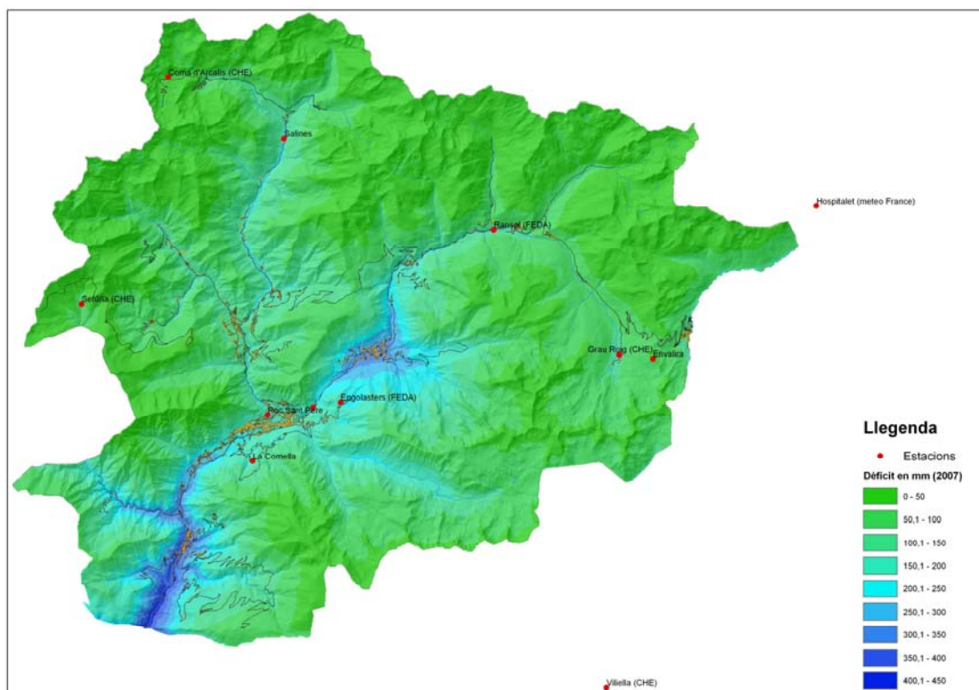
Figura 19. Mapa de distribució dels dèficits estimats per l'any 2007. R = 30 mm seguint el mètode de Thornthwaite. El mètode de càlcul ha consistit en la diferència entre ETP i ETR quan no hi ha reserva disponible.
