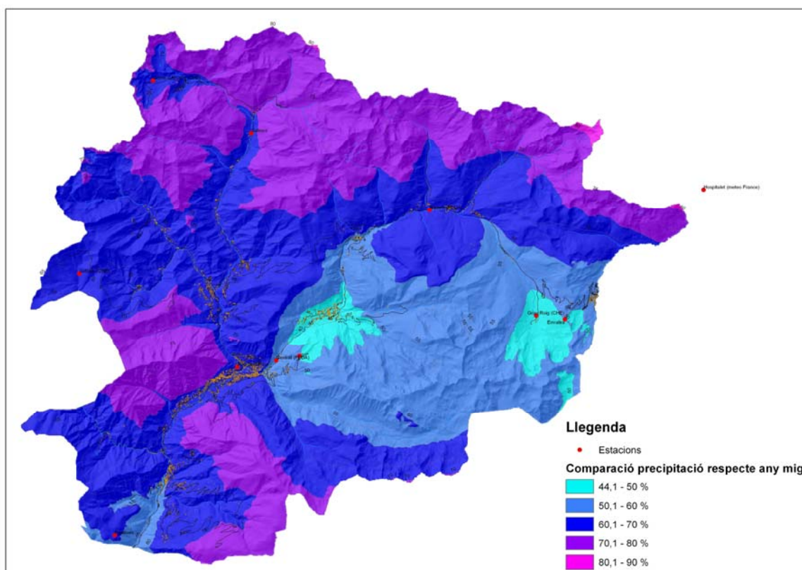
Figura 3. Mapa comparatiu de les quantitats acumulades registrades el 2007 i els corresponents valors mitjans.
