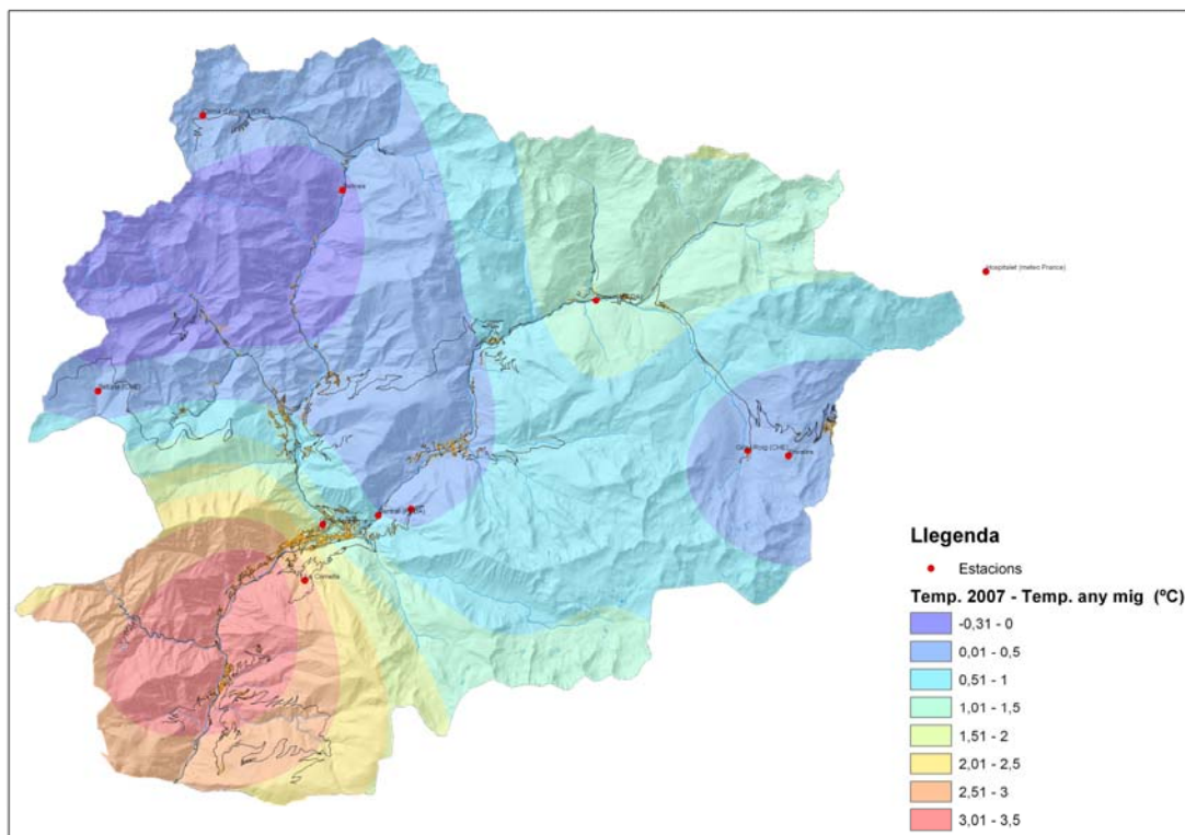
Figura 6. Mapa de les diferències de temperatura de l'any 2007 respecte la mitjana.
