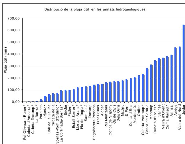
Figura 15. Gràfic de distribució de la Pluja útil
