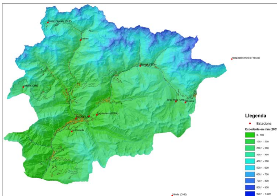
Figura 18. Mapa de distribució de la pluja útil o excedents estimats per l'any 2007. R = 30 mm seguint el mètode de Thornthwaite
