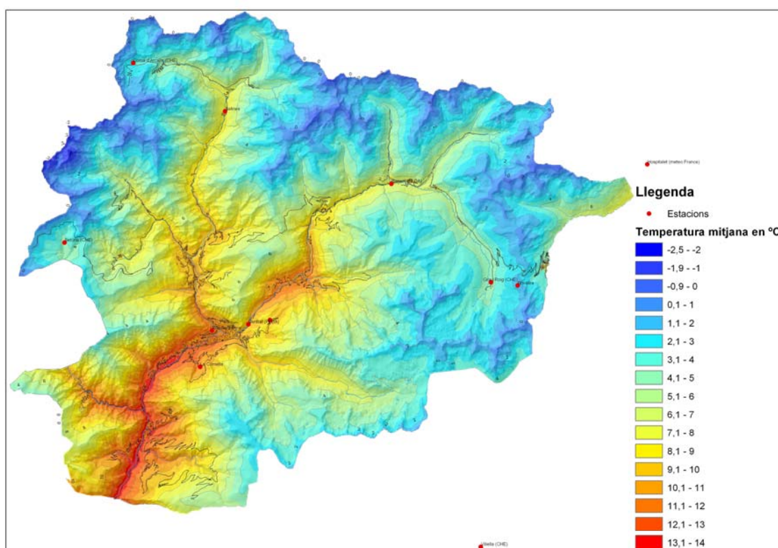
Figura 5. Mapa de distribució de les temperatures mitges del 2007
