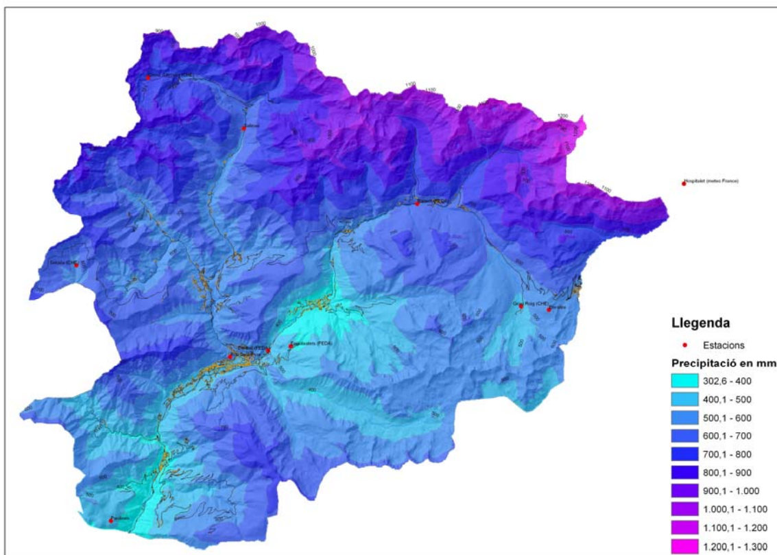
Figura 2. Mapa d'isoietes de les precipitacions acumulades el 2007.
