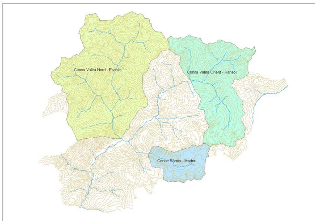
Figura 9. Mapa de situació de les conques estudiades de Valira Nord – Escalls, Conca Valira Orient Ransol i Conca Ràmio – Madriu.
