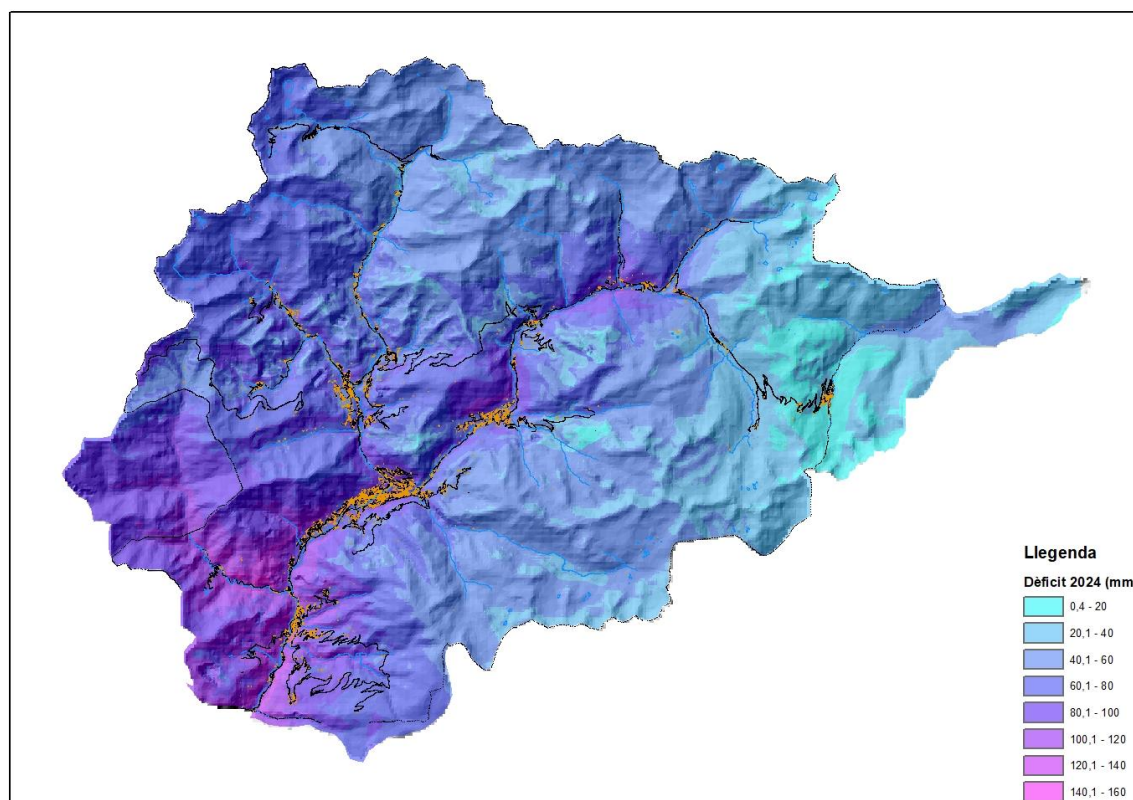
Figura 52. Mapa de distribució dels dèficits estimats per l'any 2024. R= variable, seguint el mètode de Thornthwaite El mètode de càlcul ha consistit en la diferència entre ETP i ETR quan no hi ha reserva disponible.
