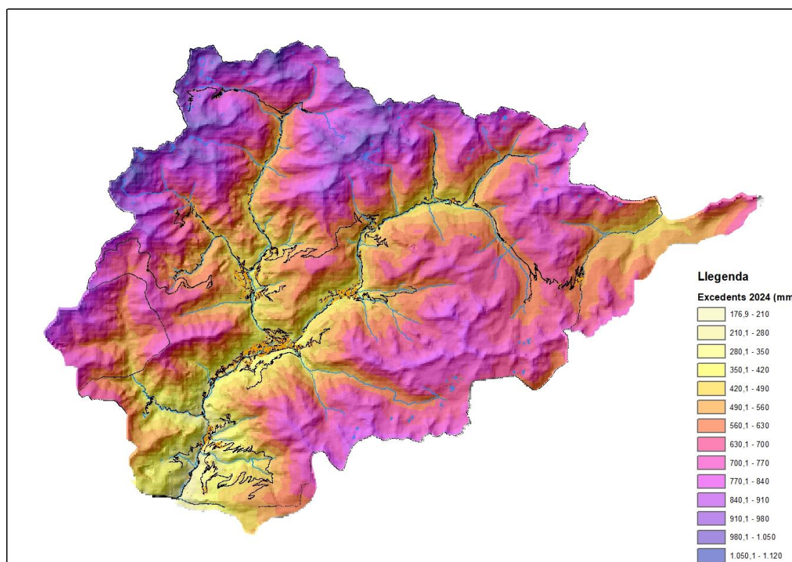
Figura 51. Mapa de distribució de la pluja útil o excedents estimats per l'any 2024
