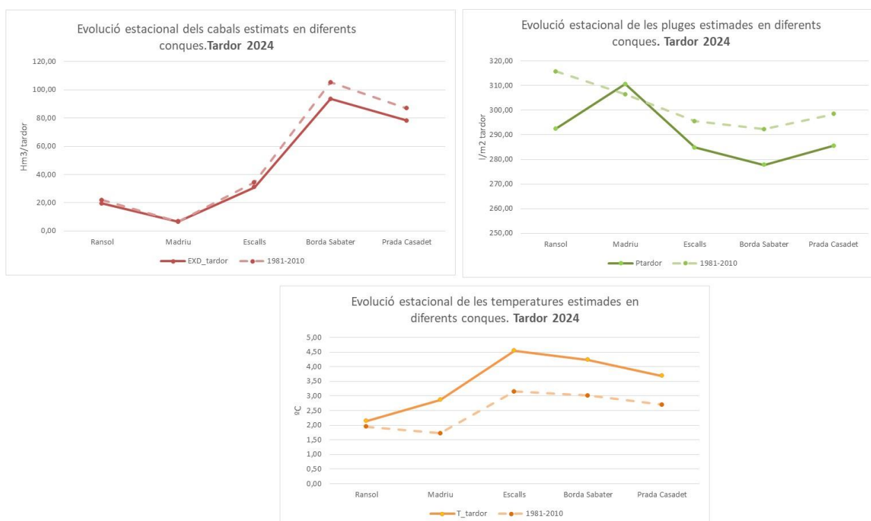
Figura 48. Anàlisi de la tardor dels cabals estimats, de les precipitacions i de la temperatura en les diferents conques.
