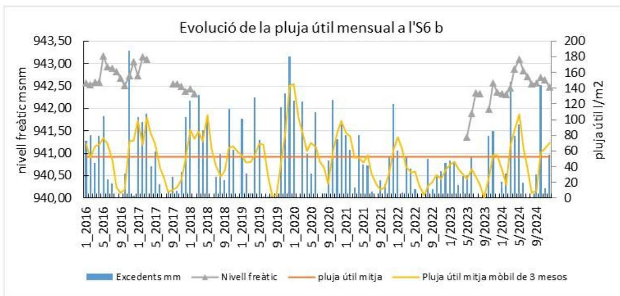
Figura 20. Evolució mensual dels nivells de l'S6b i dels excedents estimats (mitjana país)
