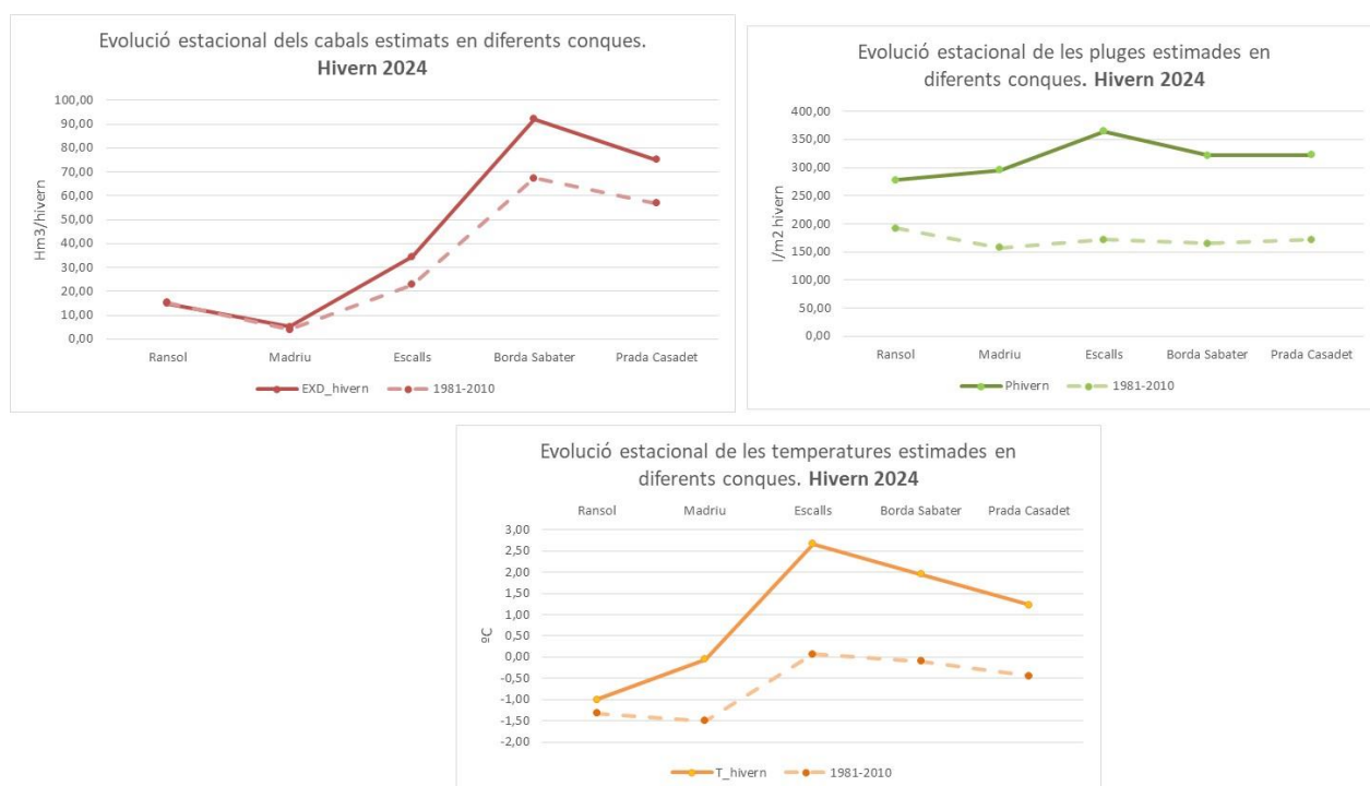
Figura 45. Anàlisi de l'hivern dels cabals estimats, de les precipitacions i de la temperatura en les diferents conques.
