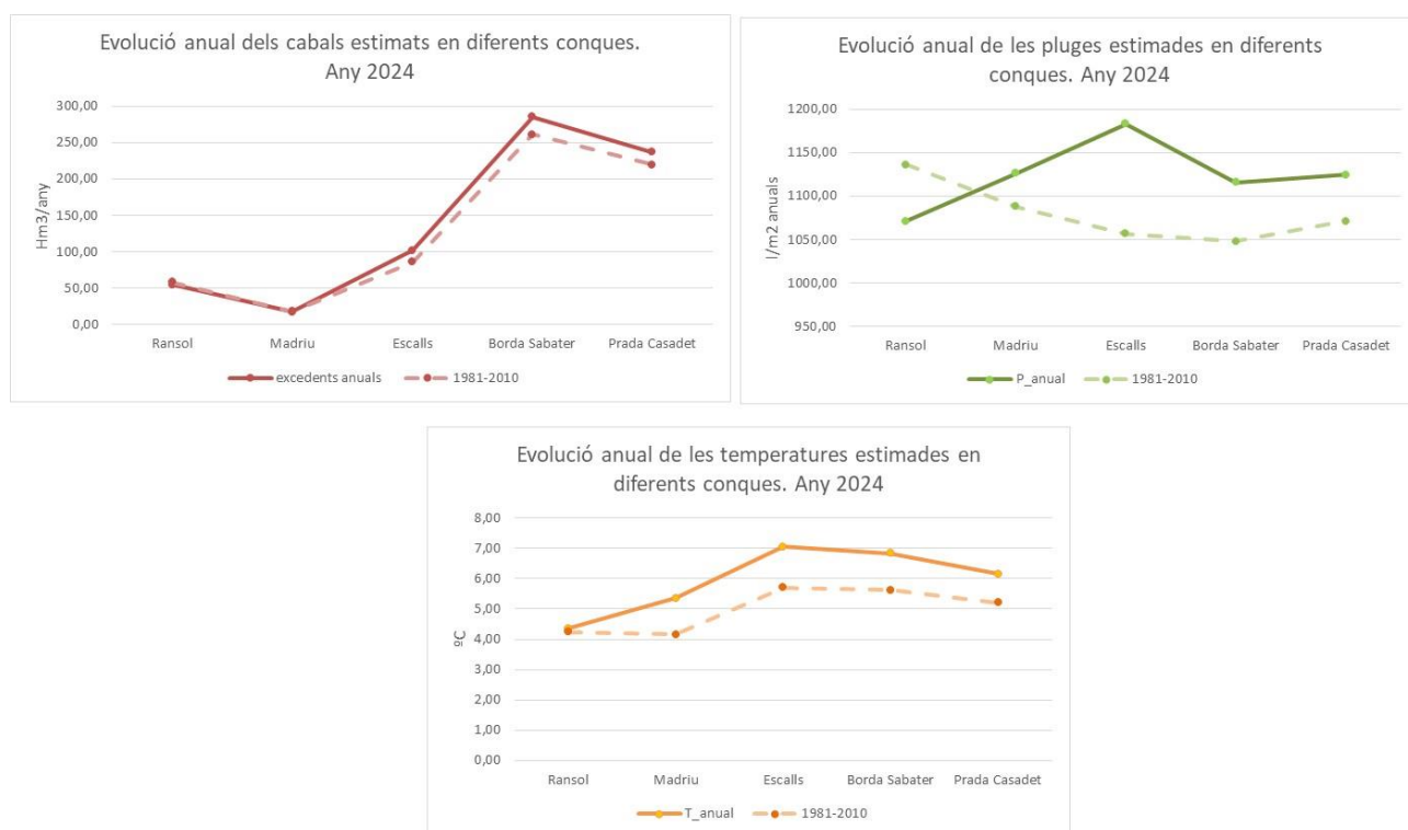
Figura 44. Anàlisi anual dels cabals estimats, de les precipitacions i de la temperatura en les diferents conques.
