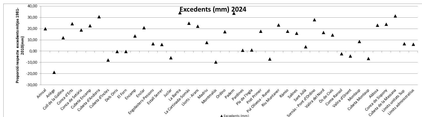
Figura 35. Gràfic de distribució dels excedents en les diferents unitats hidrogeològiques descrites en l'estudi del M.I. Govern, 2007. Si el valor mig representa el 100%, els valors del gràfic representen el percentatge per sobre o per sota la mitjana.
