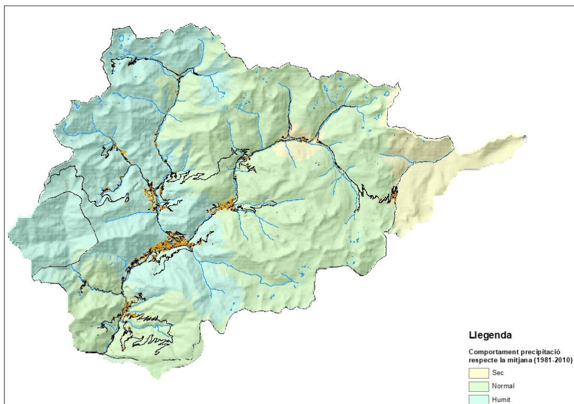
Figura 2. Mapa comparatiu de les quantitats acumulades registrades el 2024 i els corresponents valors mitjans.
