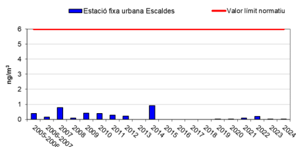
Gràfic 14. Evolució de l'arsènic (període 2005-2024)
