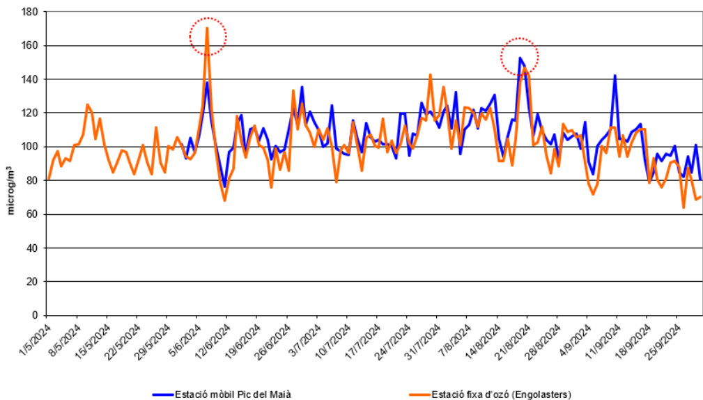
Gràfic 12: Evolució dels màxims horaris (de l'1 de maig del 2024 al 30 de setembre del 2024).
