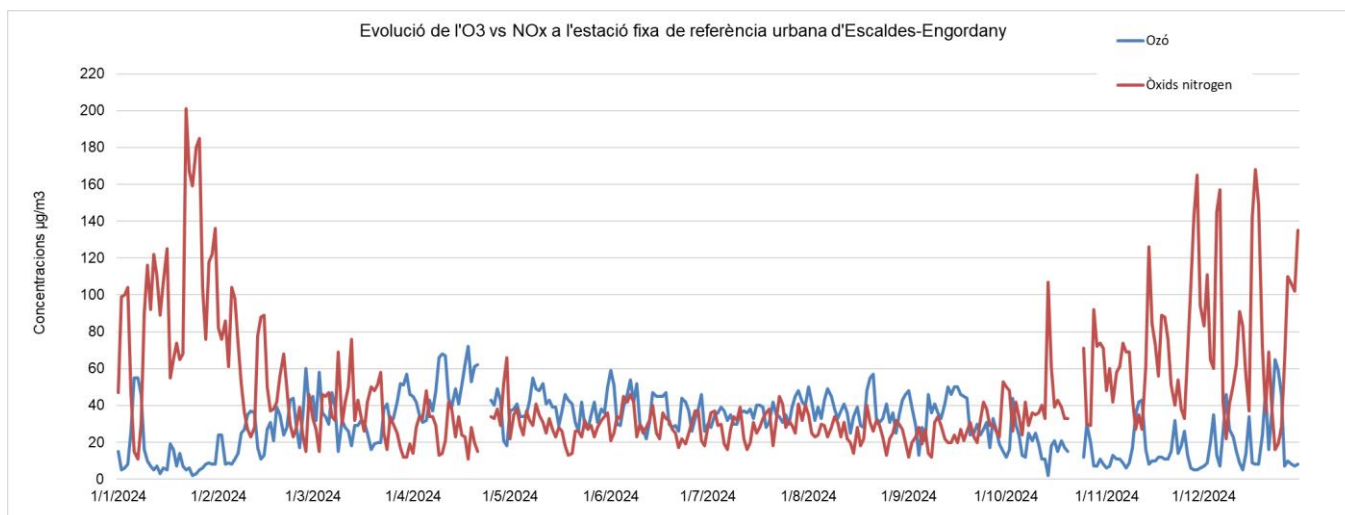
Gràfic 13: Evolució O 3 vs NO x a l'estació fixa de referència urbana d'Escaldes-Engordany. Any 2024
