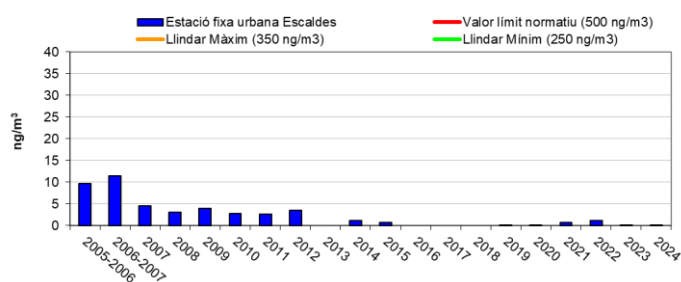
Gràfic 17. Evolució del plom (període 2005-2024)
