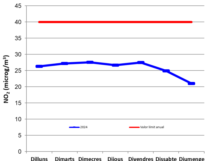
Gràfic 22. Perfil setmanal de l'NO 2 a la vall central (2024)
