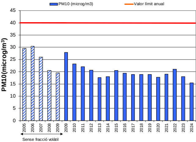
Gràfic 7. Evolució de la mitjana anual de PM 10
