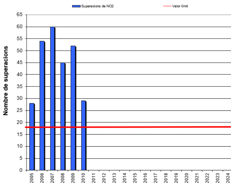
Gràfic 4. Evolució del nombre de superacions del límit horari de 200 \mu\text{g}/\text{m}^3 d' \text{NO}_2
