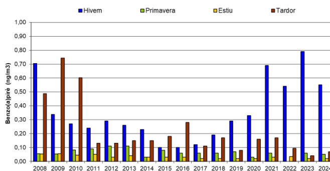
Gràfic 19. Evolució estacional del benzo(a)pirè
