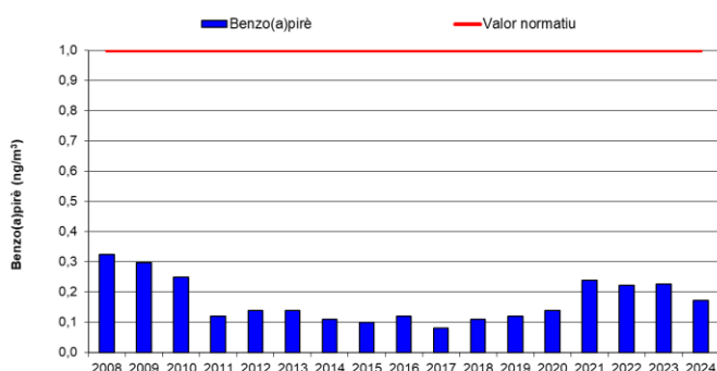
Gràfic 18. Evolució del benzo(a)pirè. Any 2008 a 2024
