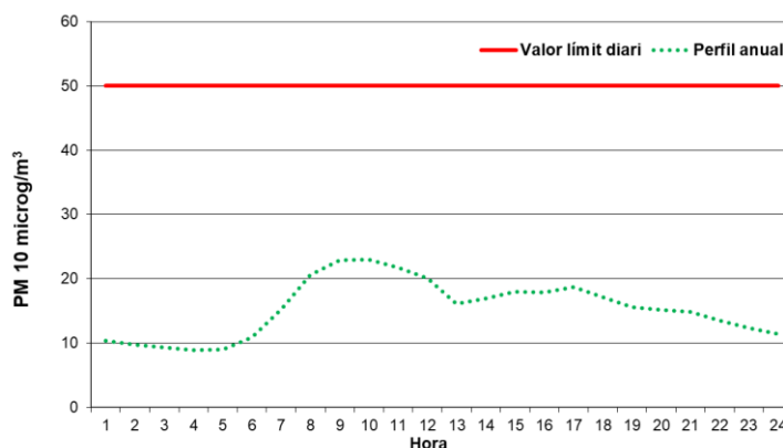
Gràfic 23. Perfil diari de partícules PM 10 a la vall central
