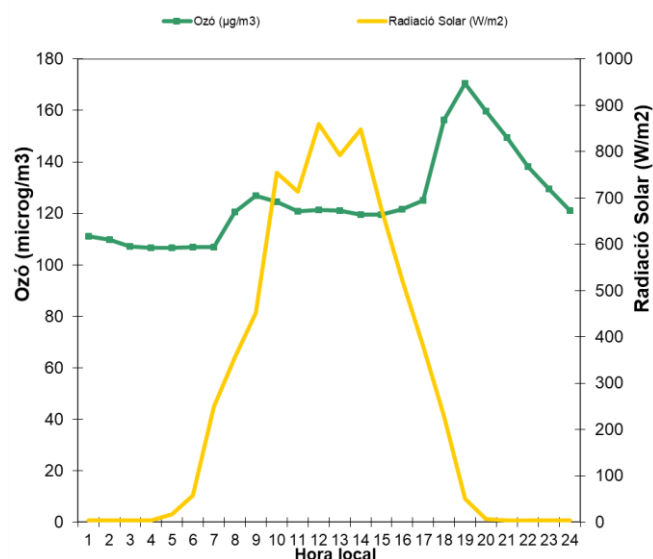
Gràfic 25. Perfil diari de l'ozó en el periurbà de la vall central (07/06/2024)
