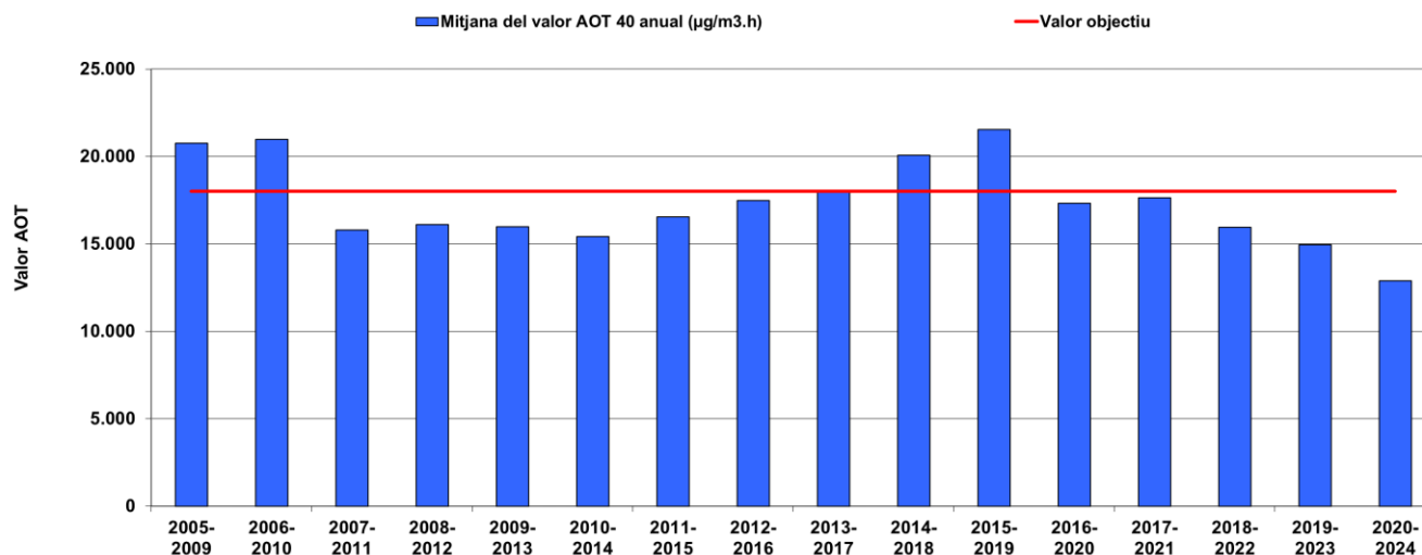
Gràfic 11. Evolució històrica dels valors de l'AOT40
