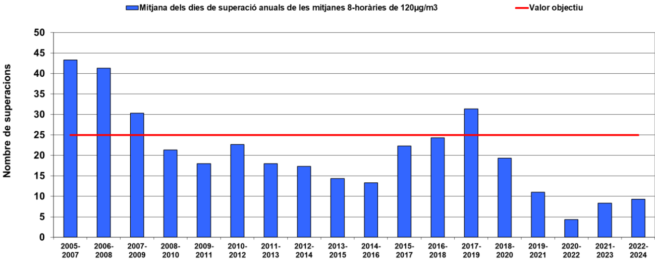
Gràfic 10. Evolució històrica del nombre de dies de superacions de 120 µg/m³.
