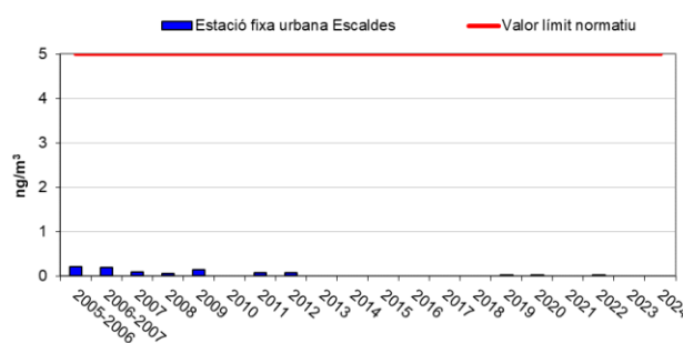
Gràfic 15. Evolució del cadmi (període 2005-2024)
