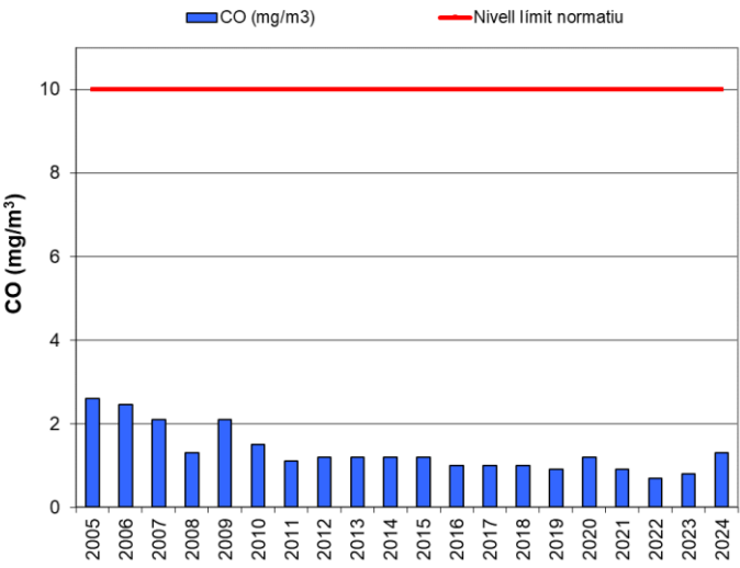
Gràfic 6. Evolució de la mitjana anual del CO
