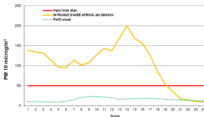
Gràfic 24. Perfil de partícules PM 10 del dia 08/04/2024 a la vall central
