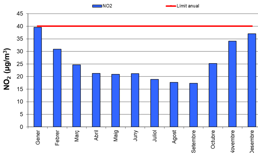
Gràfic 21. Evolució estacional de l'NO 2 a l'estació de referència urbana (any 2024).
