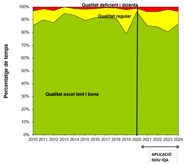
Gràfic 2. Evolució de l'IQA des de l'any 2010
