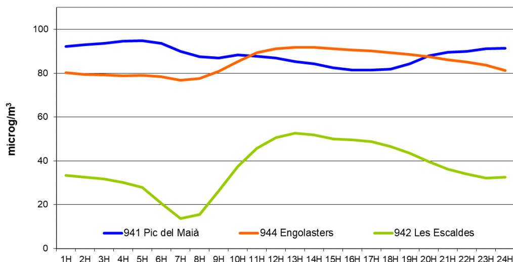
Gràfic 26: Perfil diari dels mesuraments d'ozó durant la campanya d'estiu (de l'1 de maig al 30 de setembre 2024).
