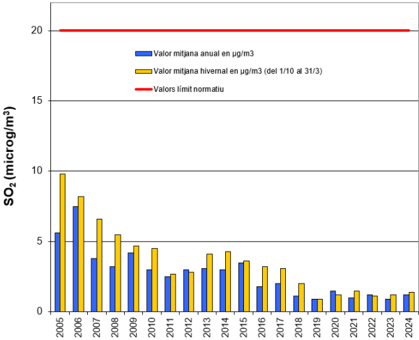
Gràfic 5. Evolució de la mitjana anual del SO 2
