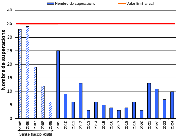
Gràfic 8. Evolució del nombre de superacions diàries
